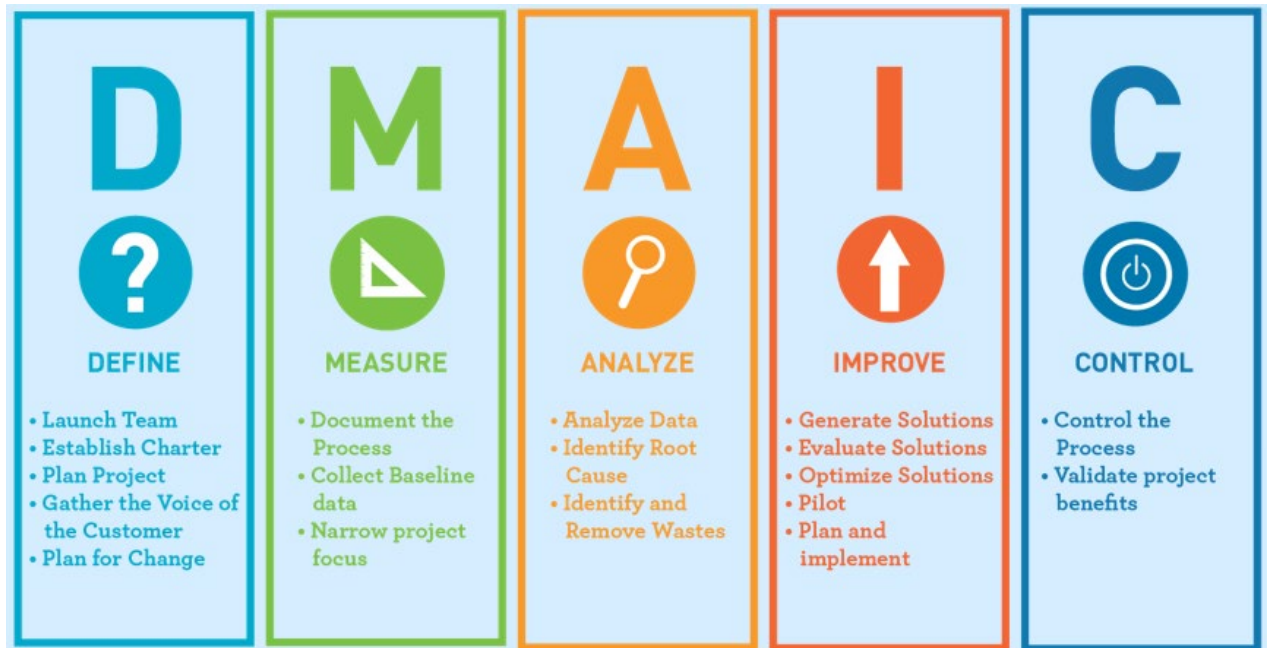
Obrázek 3. DMAIC
