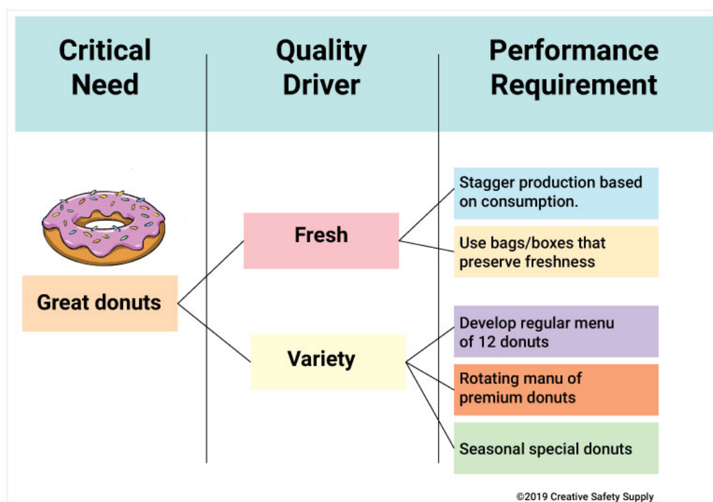
Obrázek 5. CTQ
