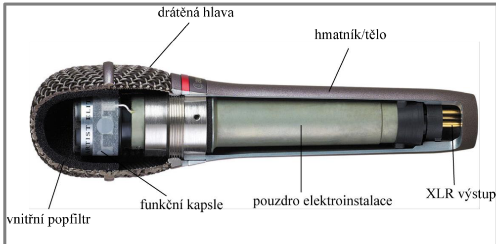
Obr. 2-5 Průřez a popis částí drátového mikrofonu AE6100 [46]
