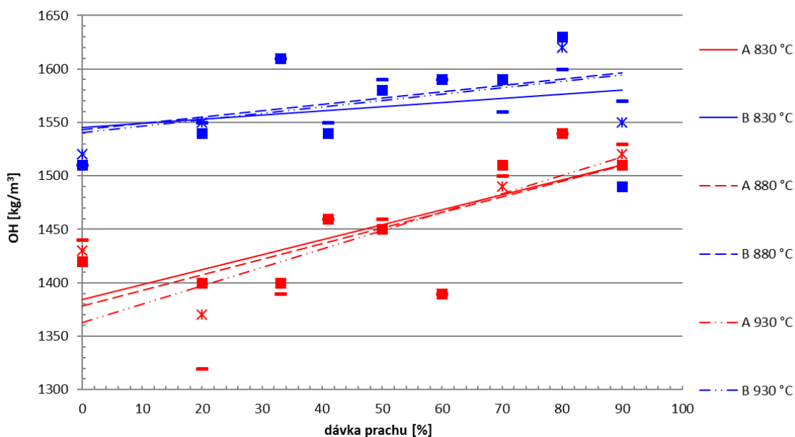
Graf 21: vliv množství cihelného prachu a teploty výpalu na objemovou hmotnost keramického střepe
