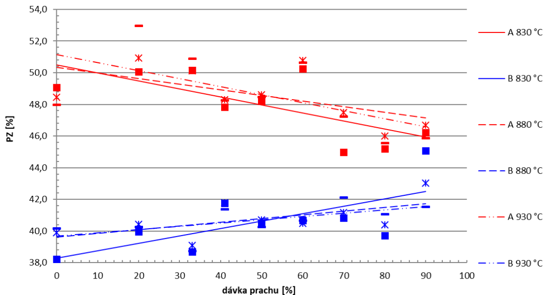
Graf 18: vliv množství cihelného prachu a teploty výpalu na zdánlivou pórovitost keramického střepe
