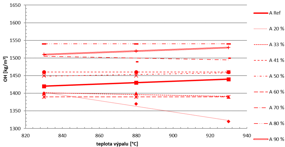
Graf 19: receptury A – vliv teploty výpalu a cihelného prachu na objemovou hmotnost keramického střepe
