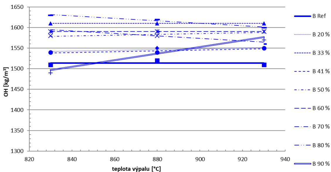
Graf 20: receptury B – vliv teploty výpalu a cihelného prachu na objemovou hmotnost keramického střepe
