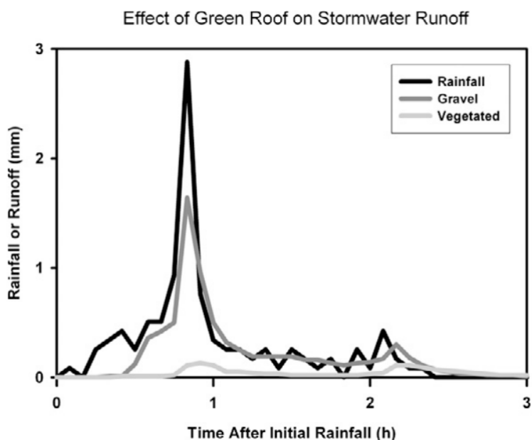
Obr. 12 – Porovnání množství (v mm) odtoku dešťových srážek (rainfall) v čase (hod.) ze střechy se štěrkovým (gravel) zásypem a ze střechy s vegetačním (vegetated) povrchem.
