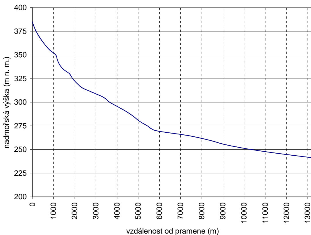
Obr. 13 Spádová křivka Dolnoněčického potoka
