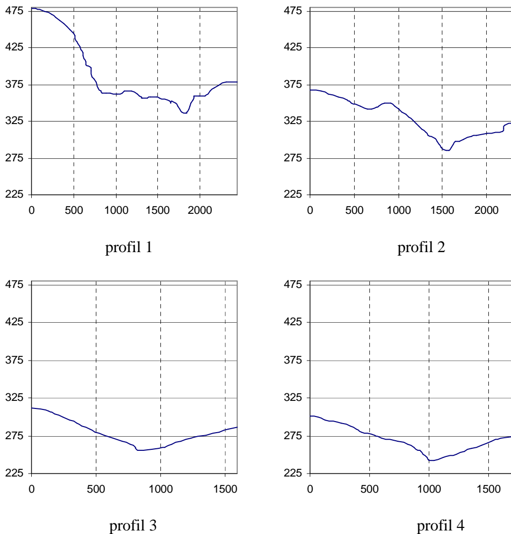
Obr. 15 Sériové profily 1, 2, 3 a 4 na Dolnonětčickém potoce
