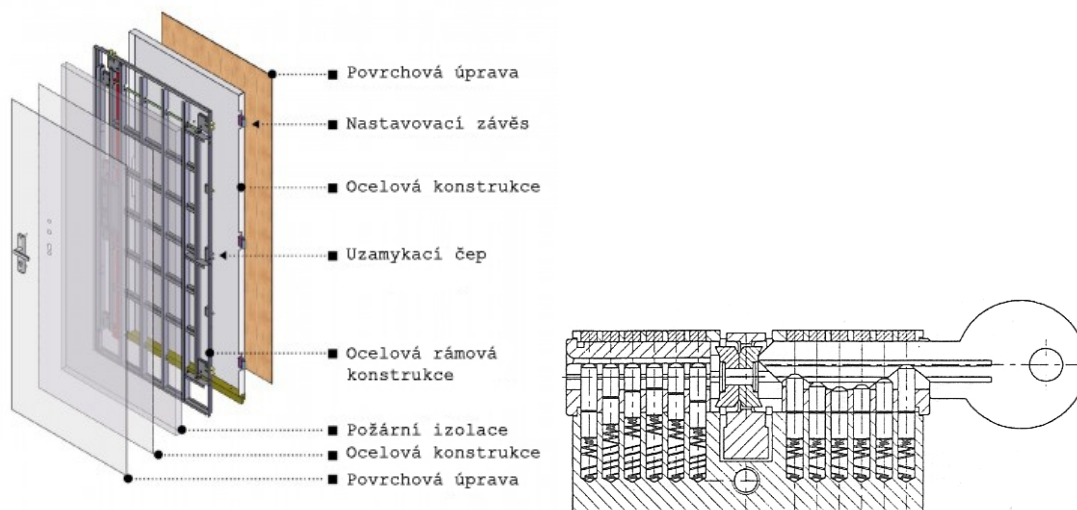
Obrázek 3.5: Bezpečnostní dveře, cylindrická vložka zámku.
