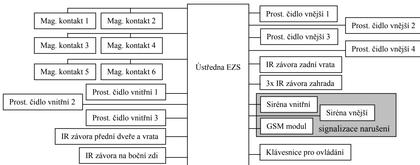
Obrázek 6.7: Blokovaný diagram návrhu systému EZS.
