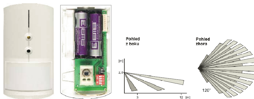
Obrázek 4.8: Jablotron JA-84P a jeho detekční charakteristika.
