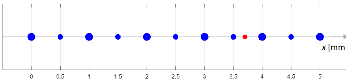
Obrázek 17: Modré puntíky reprezentují pozice na trajektorii translačního pohybu zkoumaného předmětu ve směru souřadné osy x s krokem 500 mikrometrů o celkové vzdálenosti 5 milimetrů. Pro tyto pozice předmětu jsou do databáze zaznamenány snímky struktur koherenčních zrnitostí. Červeně je vyznačena neznámá pozice předmětu, která je detekována v měřicí fázi experimentu.
