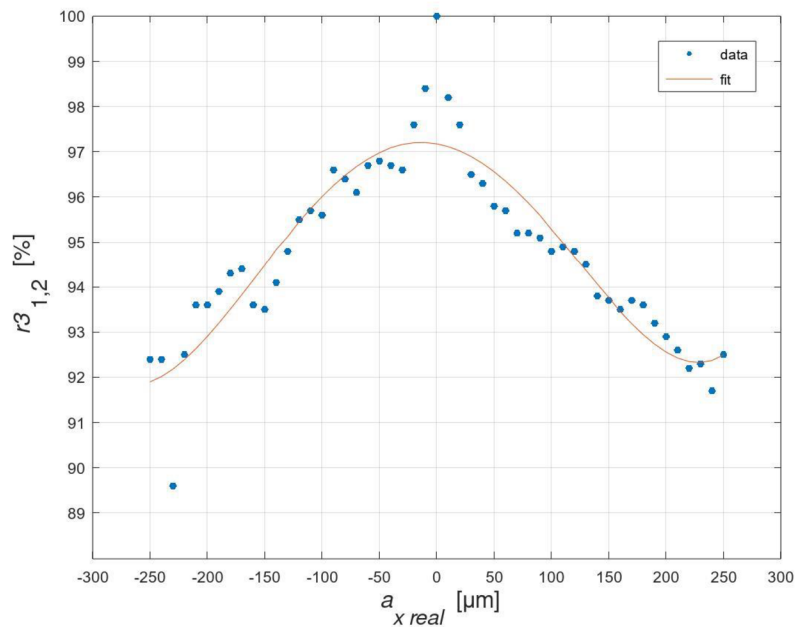
Obrázek 20: Graf závislosti stupně vzájemné korelace intenzit r_{3_{1,2}} snímků struktur koherenčních zrnitostí na reálné translaci předmětu a_{x-real} s krokem 10 mikrometrů v celkovém rozsahu translace \pm 250 mikrometrů pro třetí měření. Data jsou interpolována polynomem 4. stupně.
