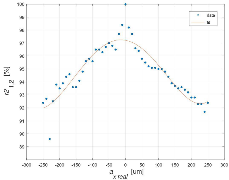
Obrázek 19: Graf závislosti stupně vzájemné korelace intenzit r_{2_{1,2}} snímků struktur koherenčních zrnitostí na reálné translaci předmětu a_{x-real} s krokem 10 mikrometrů v celkovém rozsahu translace \pm 250 mikrometrů pro druhé měření. Data jsou interpolována polynomem 4. stupně.
