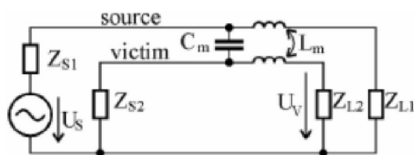
Obr. 10 – Náhradní zapojení přeslechu [10]
