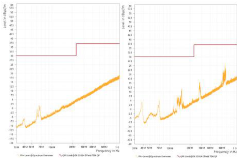
Obr. 26 – graf 2 – Porovnání vyzářování MC33063
