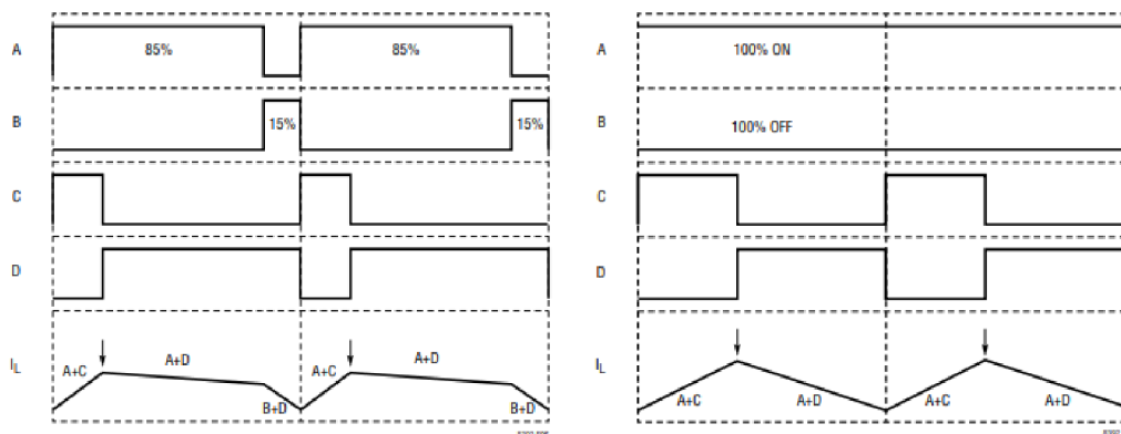
Obr. 18 – Časový diagram spínačů v oblasti boost
