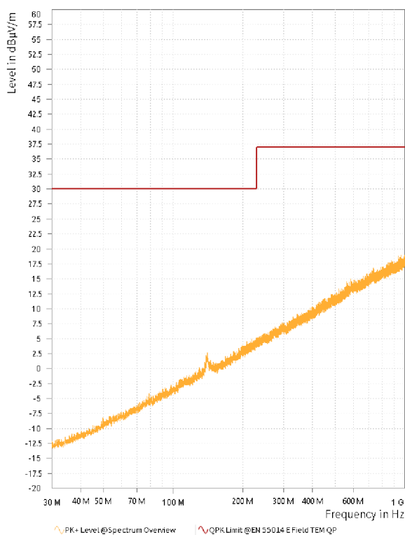
Obr. 36 – graf 8 – Měření obvodu LM317 ve vyzařovací komoře
