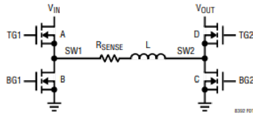
Obr. 16 – Náhradní zapojení spínací části obvodu LT8392 [9]
