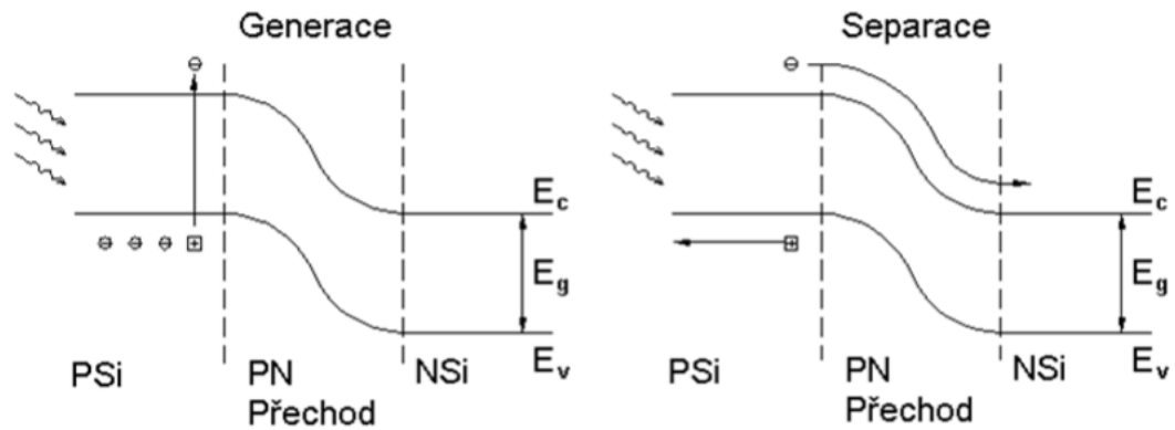
Obrázek 18. Znáornění principu fotoelektrického jevu[14]
