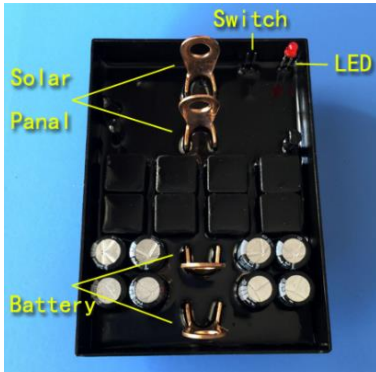
Obrázek 40. Regulátor
