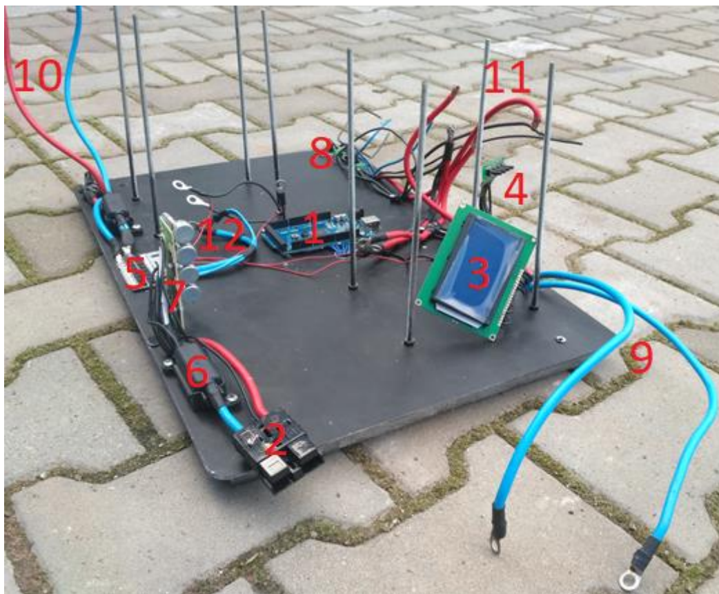
Obrázek 63. Přízemní patro elektrárny
