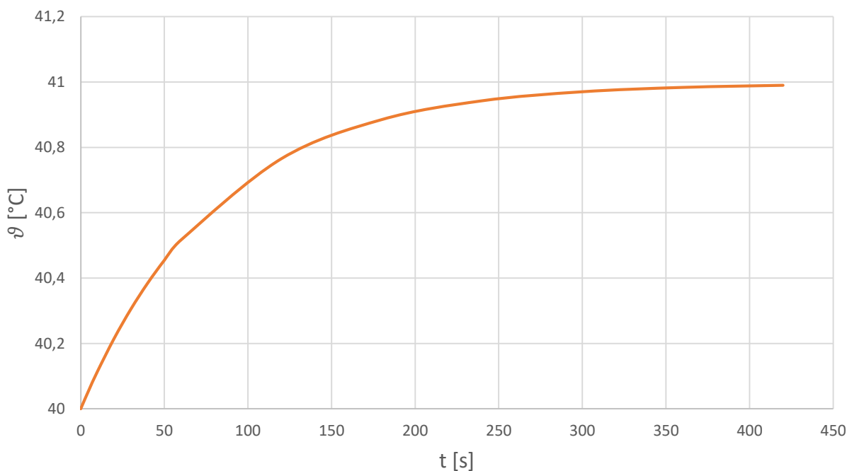
Obrázek 49. Průběh oteplení kabelu 2 \times 2,5 \text{ mm}^2 při proudem 5,4A a teplotě okolí 40^\circ\text{C}
