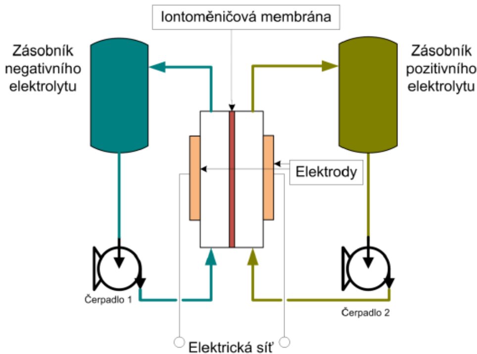
Obrázek 35. Princip průtokové baterie [13]
