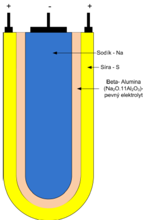
Obrázek 34. Schéma sodíkové baterie. [13]
