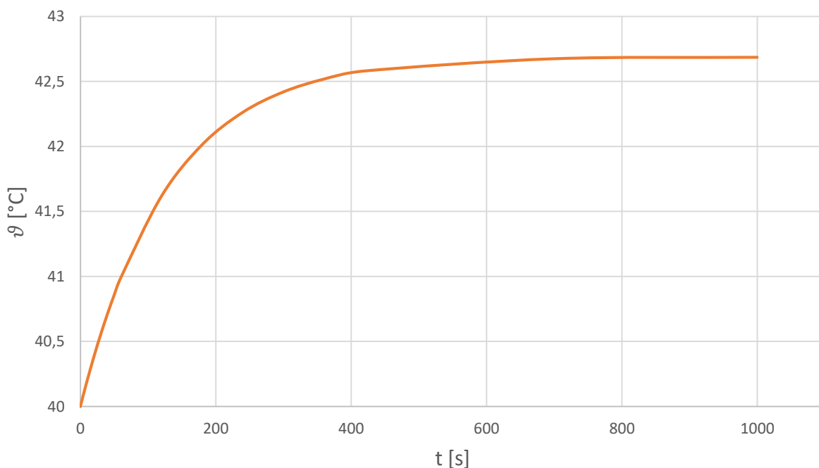
Obrázek 50. . Průběh oteplení vodiče 1 \times 10 \text{ mm}^2 při průchodu proudem 27A a teplotě okolí 40^\circ\text{C}
