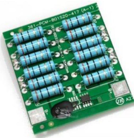
Obrázek 57. Balancovací modul pro LiFePo4
