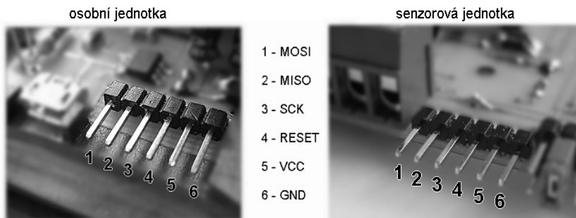
Obr. 4: Umístění vývodů nutných k naprogramování MCU
