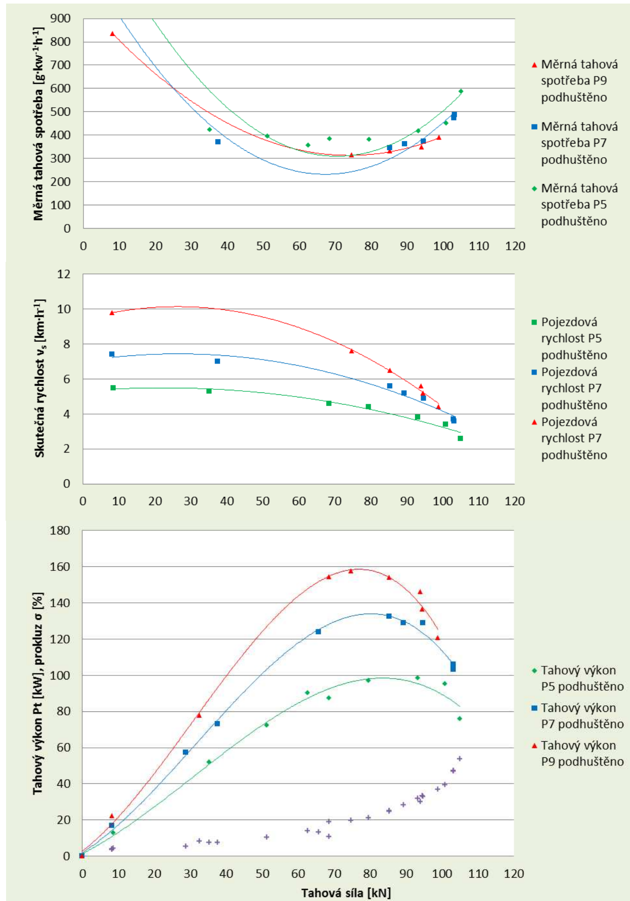
Příloha 1 Tahová charakteristika traktoru JD 8320R při tlaku huštění pneumatik 160/140 kPa
