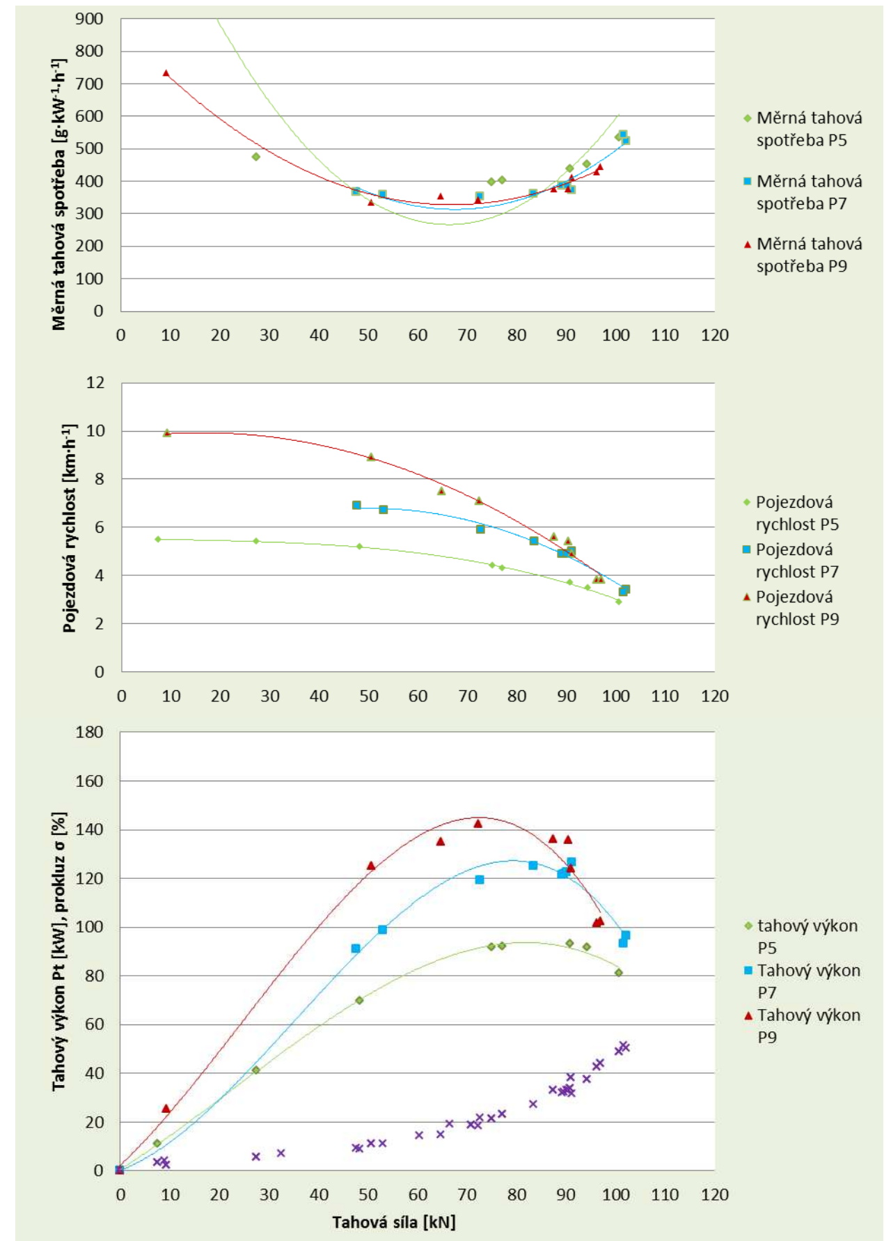
Příloha 2 Tahová charakteristika traktoru JD 8320R při tlaku huštění pneumatik 120/100 kPa
