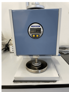
Obr. 6. Tloušťkoměr MESDAN
