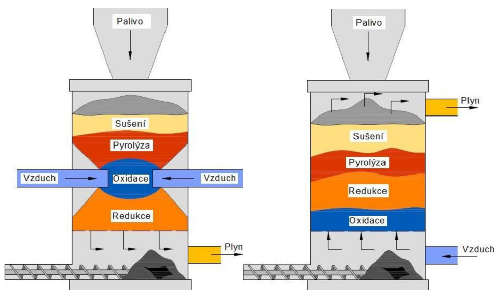
Obrázek 3 Schéma dvou různých typů sesuvných generátorů (souproutý a protiproutý reaktor)
