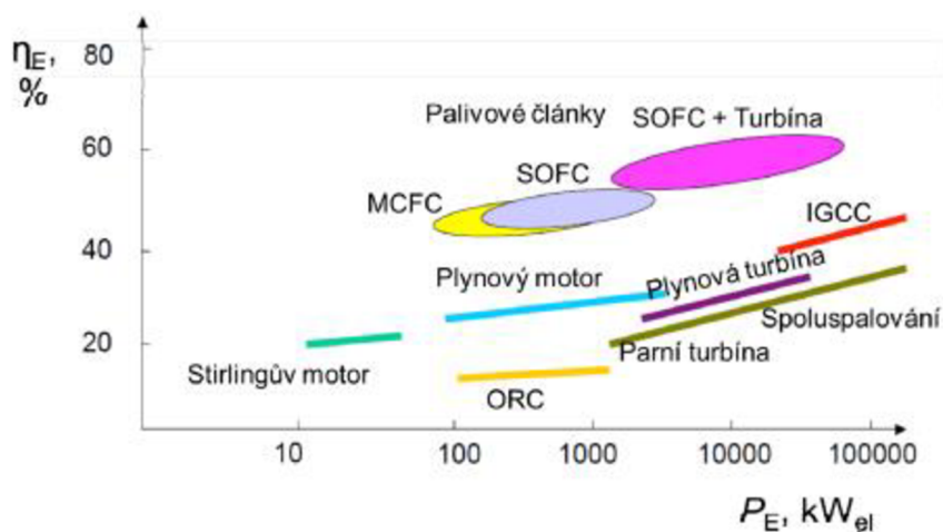
Obrázek 15 Přehled jednotlivých technologií pro kogenerační výrobu elektřiny a tepla spolu s jejich orientační účinností ( \eta_E ) a výkonovým měřítkem
