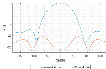
Směrová charakteristika v H-rovině na kmitočtu 400 MHz (rozdělené složky (optimalizovaná anténa))
