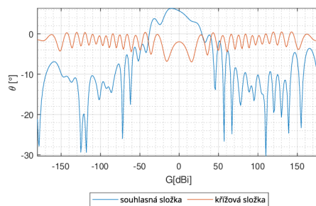
Směrová charakteristika v H-rovině na kmitočtu 3000 MHz (rozdělené složky) (anténa s krytem)
