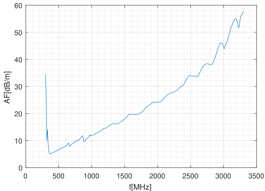
Obr. 2.13: Závislost anténního faktoru na kmitočtu - anténa s krytem
