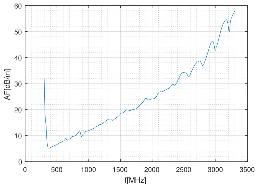
Obr. 2.18: Závislost anténního faktoru na kmitočtu - anténa s krytem a úchytem
