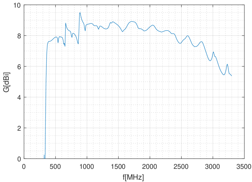
Obr. 2.12: Závislost zisku na kmitočtu - anténa s krytem
