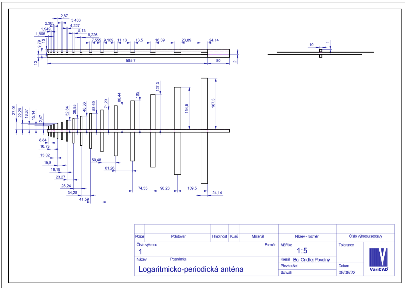
Obr. G.1: Výkres antény
