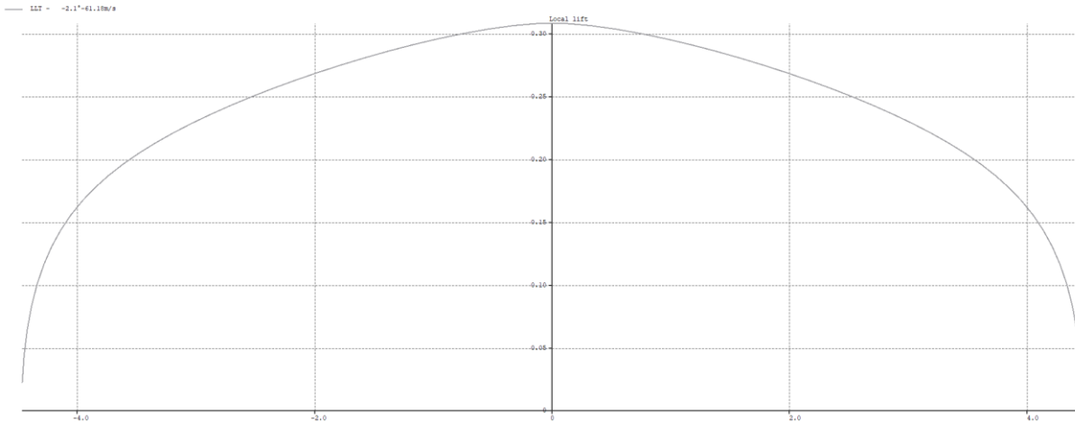
Obrázok 38 Graf rozloženia vztlaku po krídle c_l c / c_{mac} .
