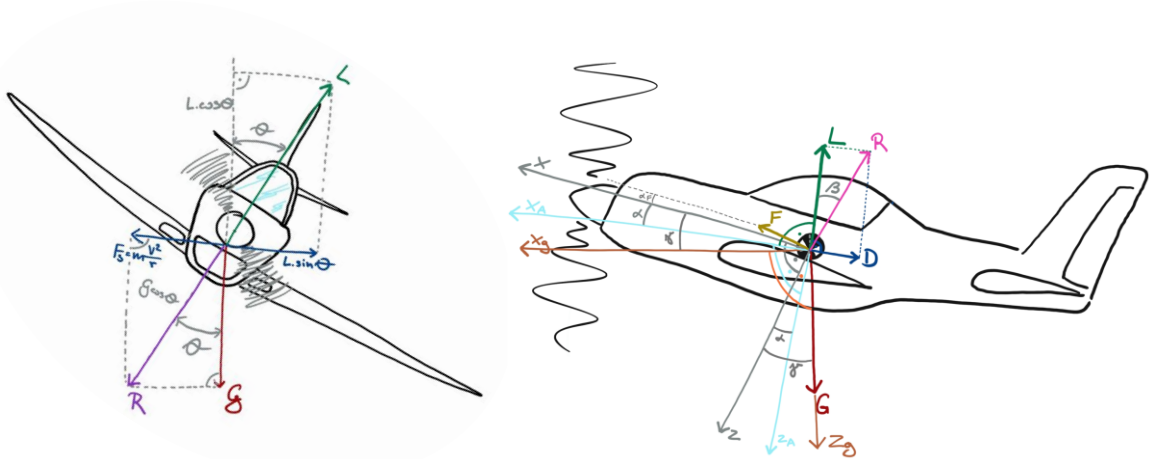
Obrázok 12 Znáznorenie uhlov a vektorov síl voči súradnicovým systémom (správna zatáčka a klopenie). [12] (upravené autorom)
