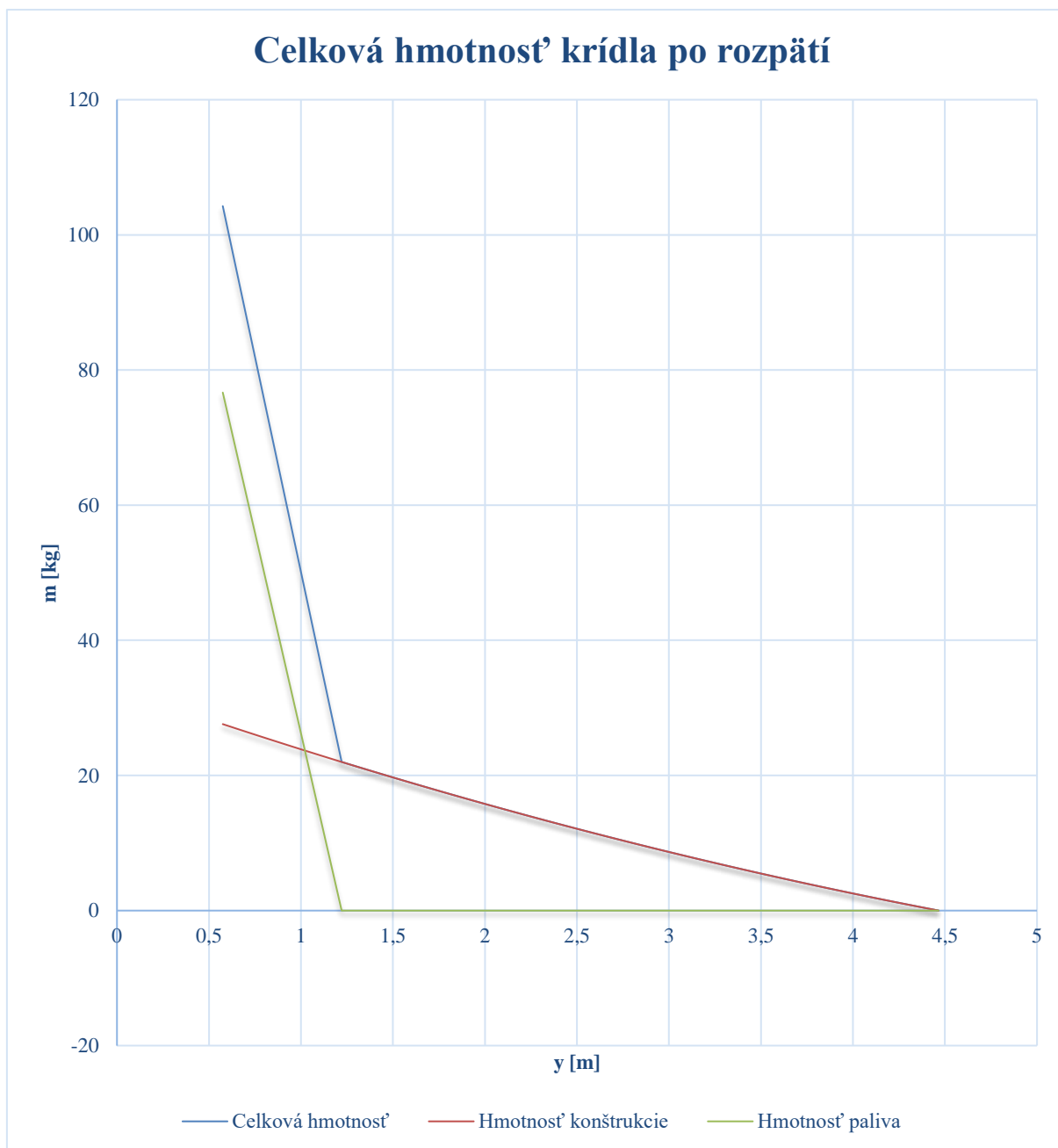
Graf 5 Celková hmotnosť krídla po rozpätí ako súčet hmotností konštrukcie a paliva.
