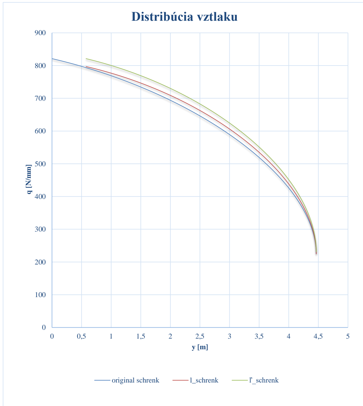
Graf 4 Rozloženie vztľaku po krídle.
