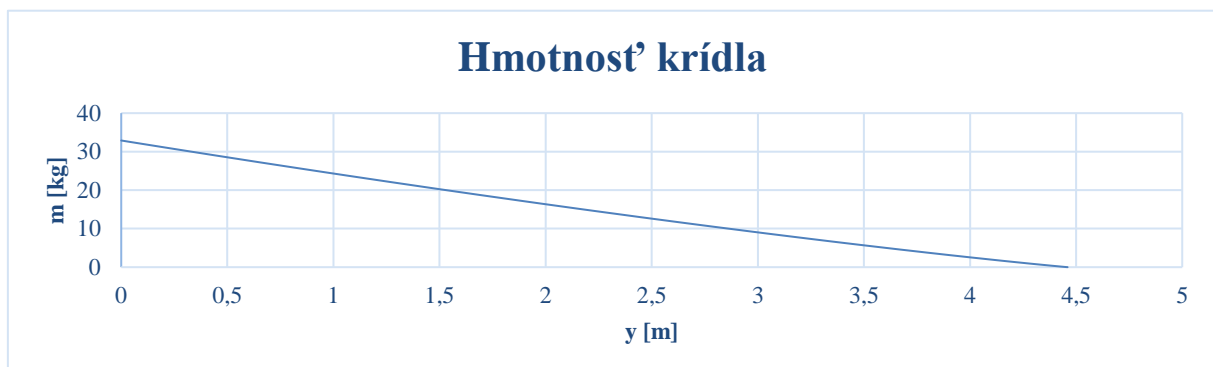
Graf 12 Priebeh hmotnosti krídla po rozpätí.
