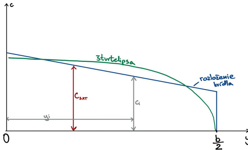
Obrázok 6 Graf rozloženia krídla a štvrtelipsy.
