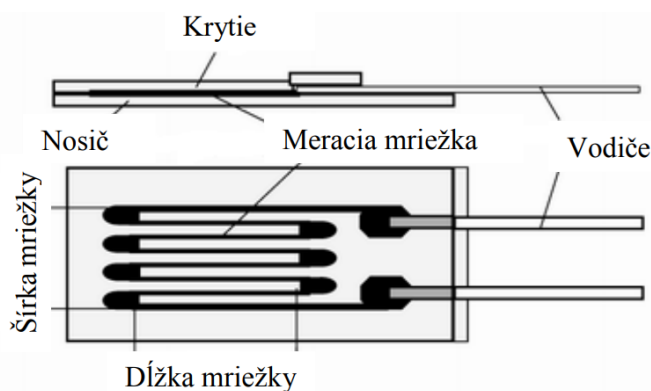
Obrázok 42 Fóliový tenzometer. [21]
