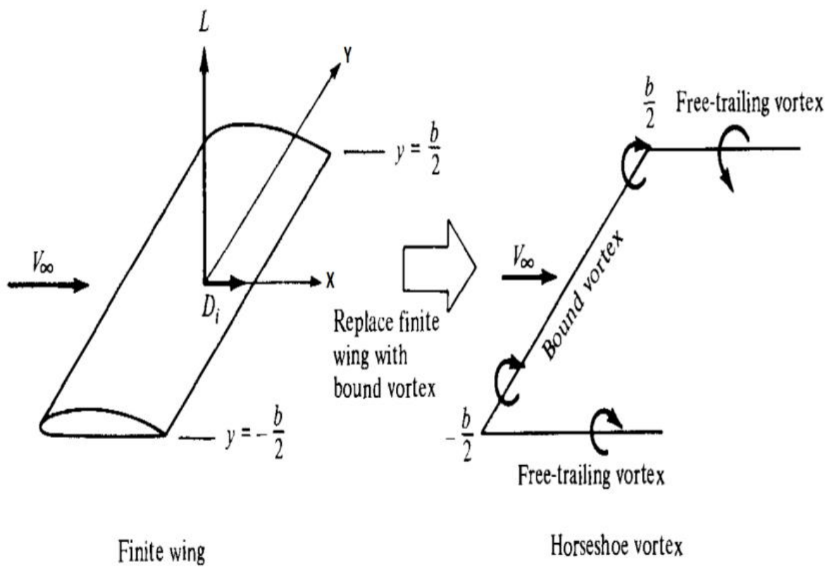
Obrázok 25 Vír s konštantnou silou \Gamma reprezentujúci krídlo. [17]
