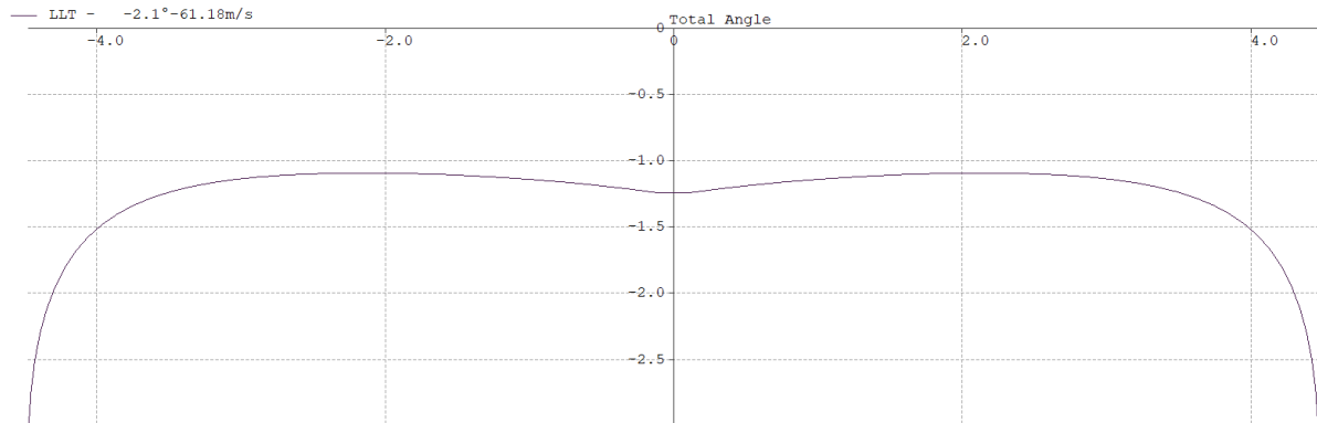
Obrázok 39 Graf lokálneho uhlu nábehu \alpha_{eff} .
