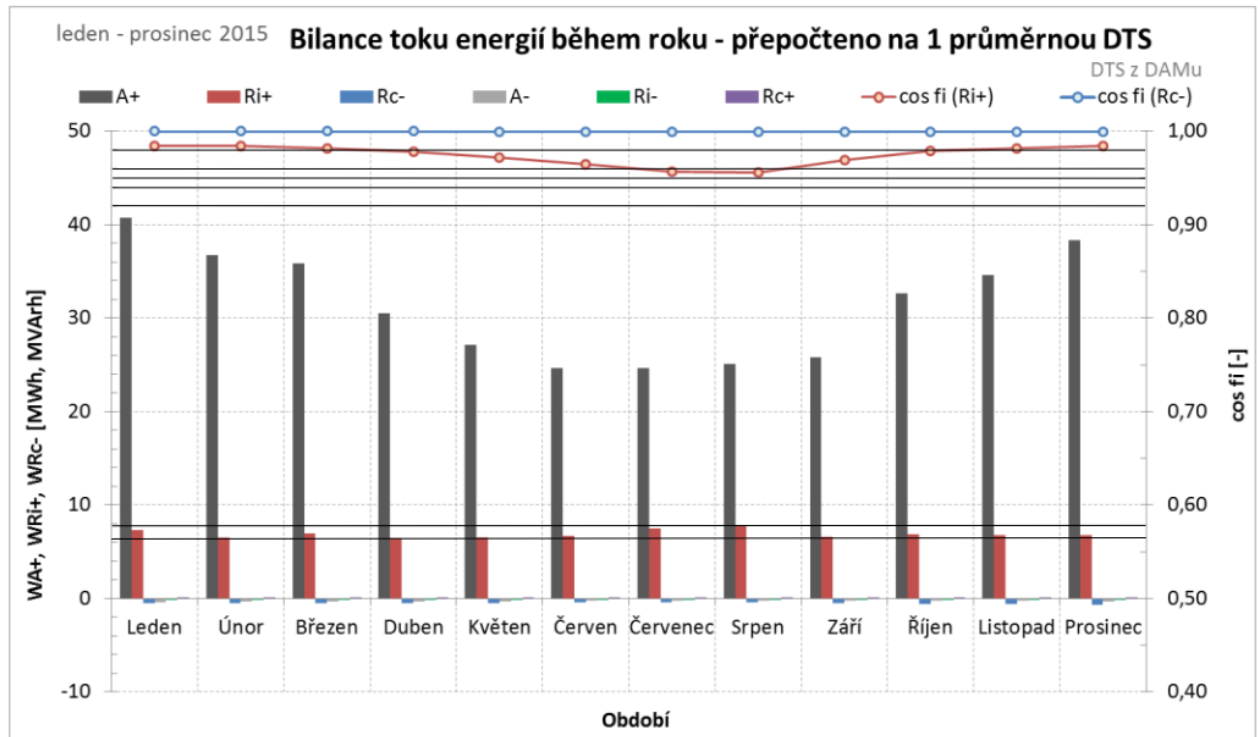
Obr. 3-9 Toky energií přepočteny na průměrnou DTS (převzato z [9])
