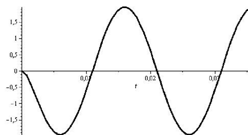
Obrázek 10: Časový průběh elektrického proudu i_2(t)A
