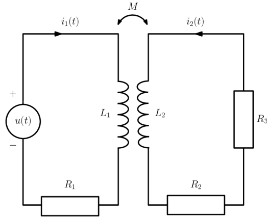
Obrázek 8: Schéma uvažovaného elektrického obvodu
