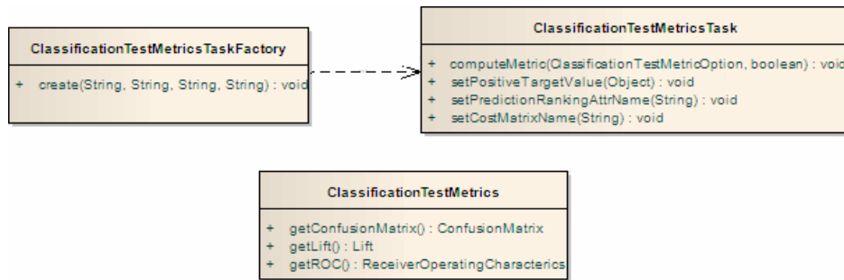
Obr. 5.3: Třídy pro vytvoření testovacích metrik
