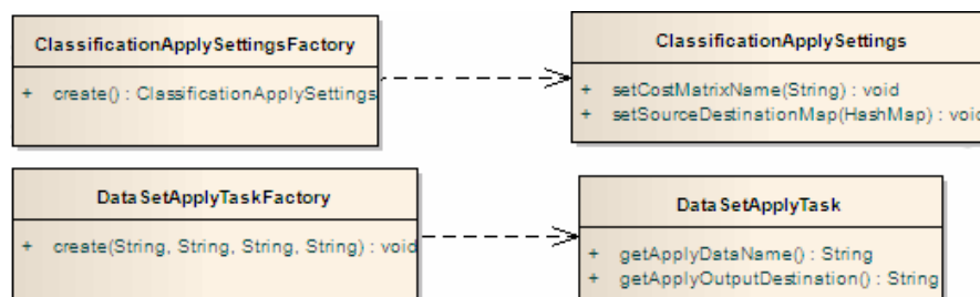
Obr. 5.4: Třídy pro aplikaci
