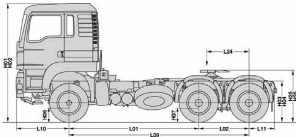
Obrázek 8 Tahač MAN [14]
