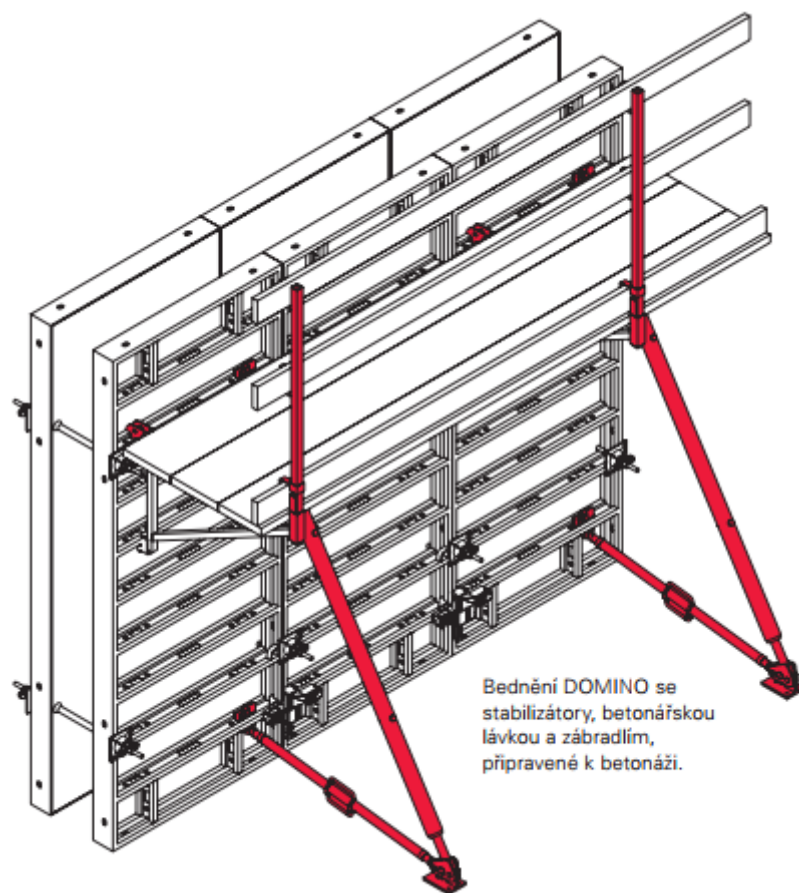
Obrázek 21 Stěnové bednění [26]
