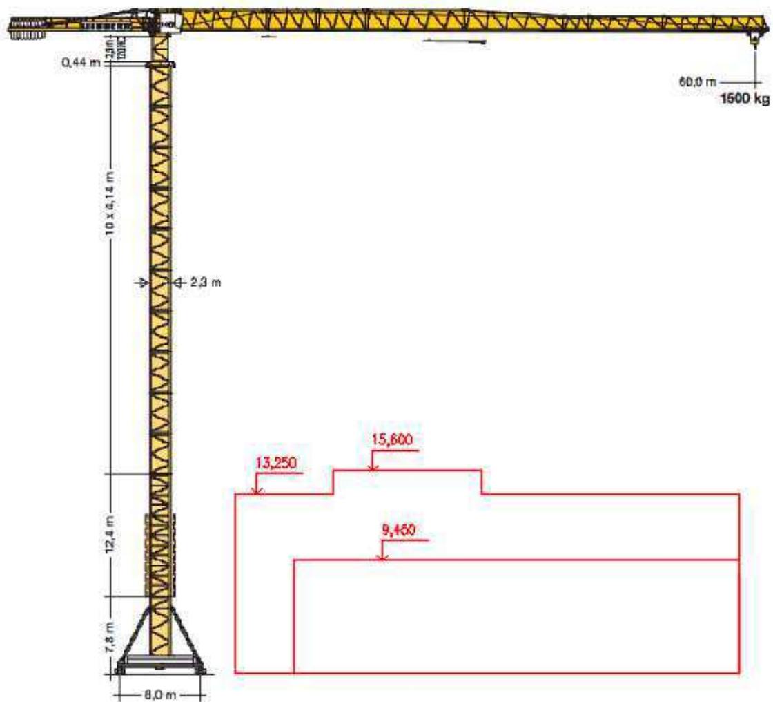
Obrázek 14 Rozměry věžového jeřábu [20]
