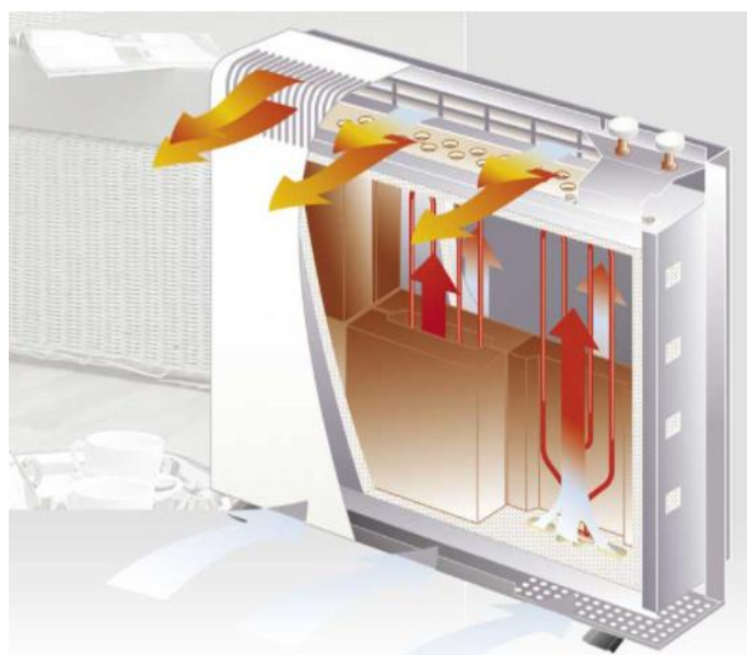
Obr. 3.3 Akumulační kamna [68]
