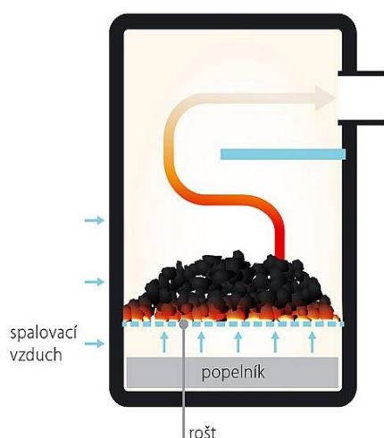
Obr. 1.5 Prohořivací kotel [58]
