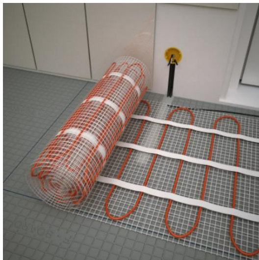
Obr. 3.1 Topné rohože [62]
