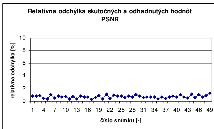
Obr. 23 Retatívna odchýlka skutočných a odhadnutých hodnôt PSNR pre videosekvenciu „bridge_close_cif“
