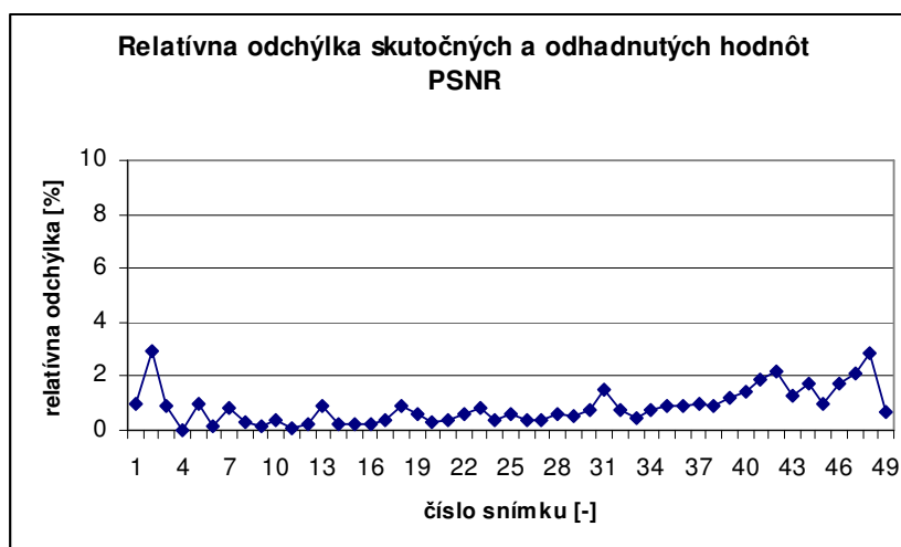
Obr. 24 Relativná odchýlka skutočných a odhadnutých hodnôt PSNR pre videosekvenciu „coastguard_cif“
