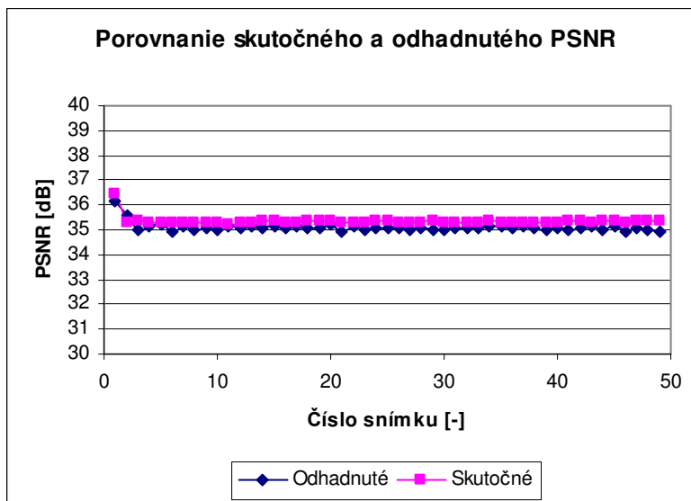
Obr. 20 Porovnanie skutočného a odhadnutého PSNR pre videosekvenciu „bridge_close_cif“
