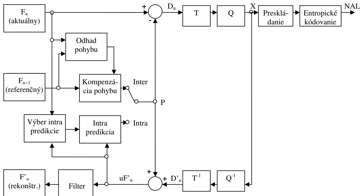
Obr. 1 H.264 Enkodér.
