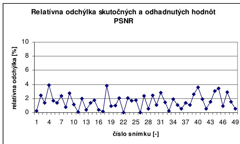
Obr. 22 Retatívna odchýlka skutočných a odhadnutých hodnôt PSNR pre videosekvenciu „flower_cif“
