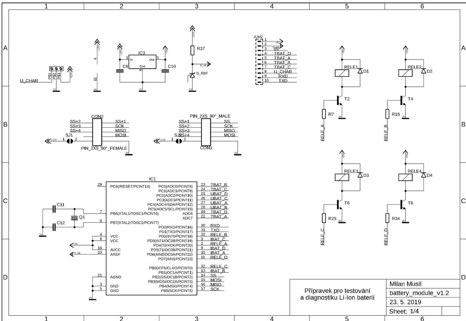
Příloha 3 Modul baterií
