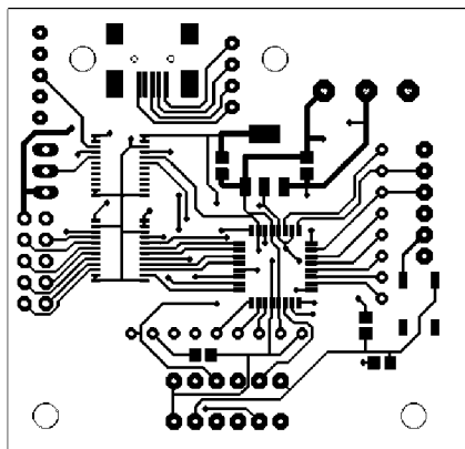
Příloha 7 Top strana desky řídicího modulu
