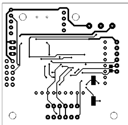
Příloha 8 Bottom strana desky řídicího modulu
