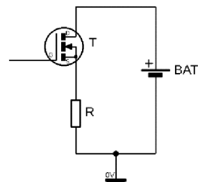
Obr. 3.6 Vybíjení článku
