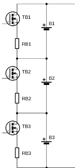
Obr. 2.2 Vyvažovač
