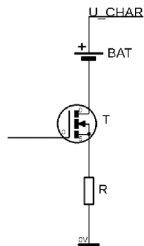
Obr. 3.5 Nabíjení článku
