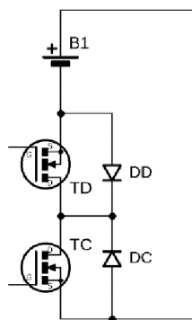
Obr. 2.1 Odpojení baterie
