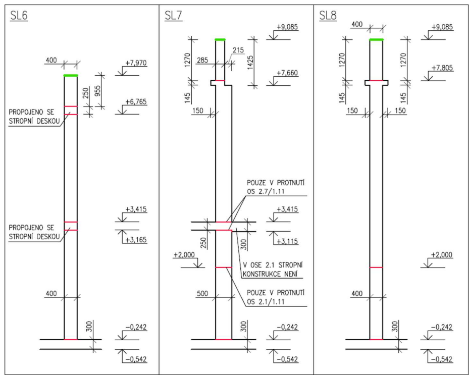
Obrázek 15 - pracovní spáry sloupů SL6 - SL8
