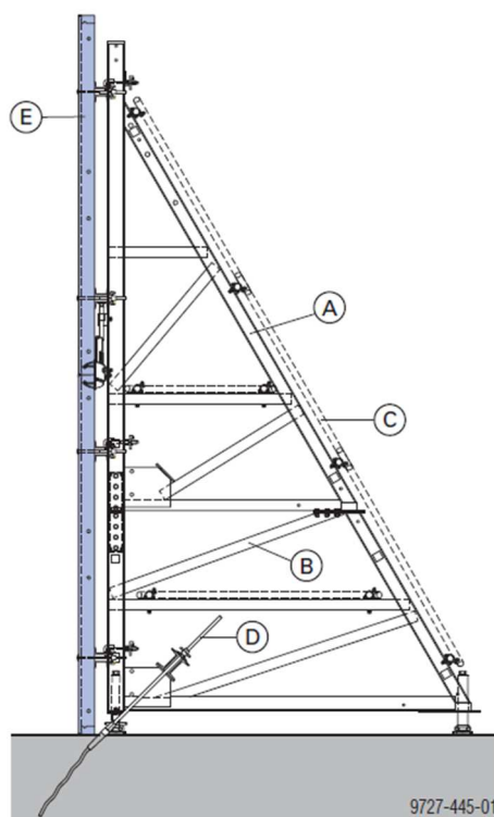
Obrázek 18 - jednostranné bednění stěn (ilustrativní foto) [7]
