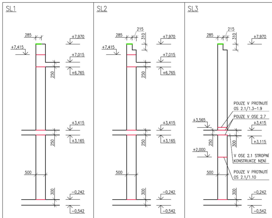
Obrázek 13 - pracovní spáry sloupů SL1 - SL3
