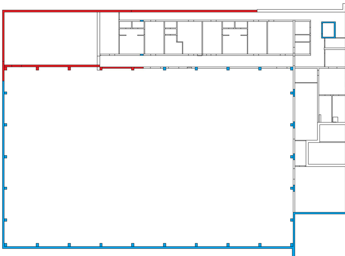
Obrázek 11 - schéma rozdělení provádění ŽB konstrukcí 1.NP
