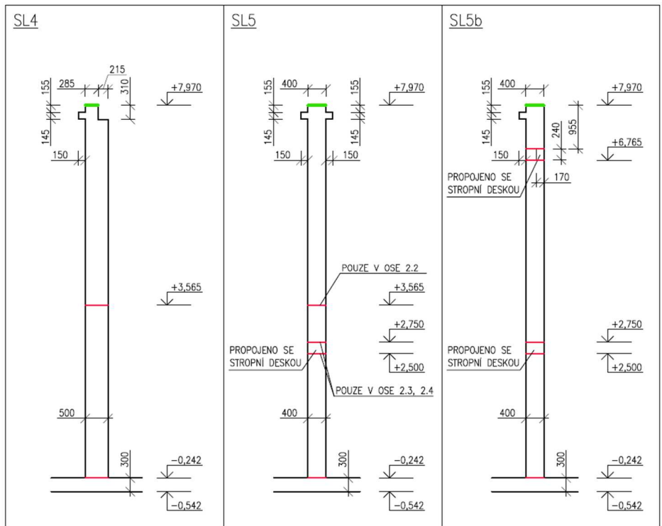
Obrázek 14 - pracovní spáry sloupů SL4 - SL5b
