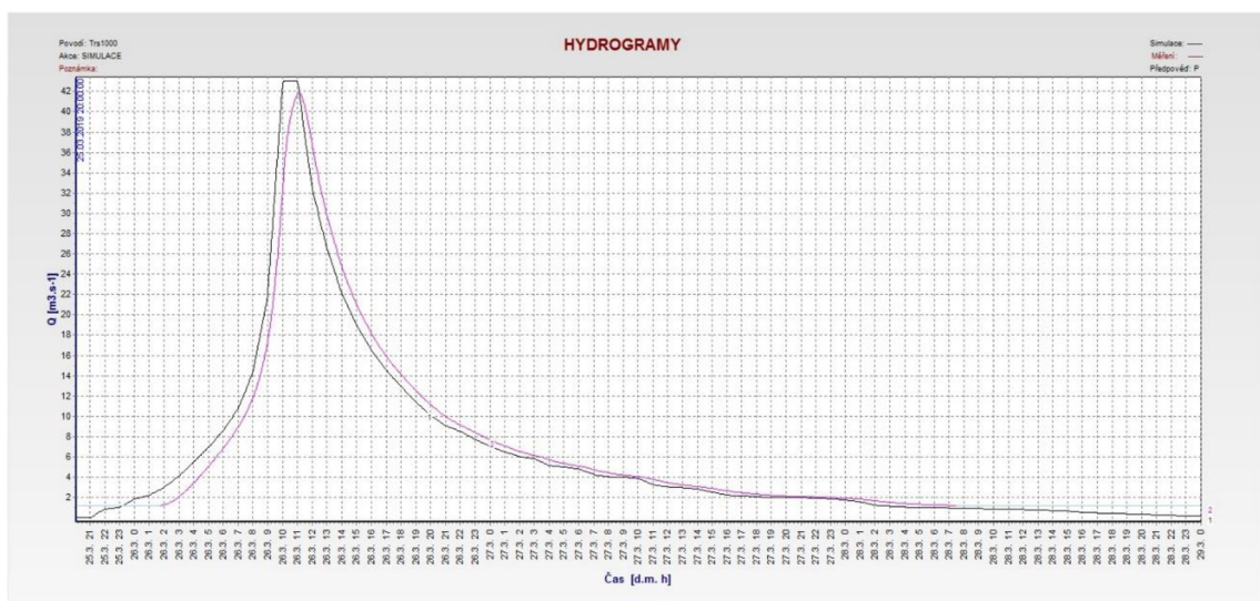
Obr. 13 Transformace povodně Q_{1000} pro H_{přel,hm} = 287,90 \text{ m n.m.}
