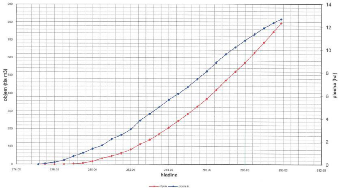
Graf 1 Batygrafické čáry nádrže Tršice [3]
