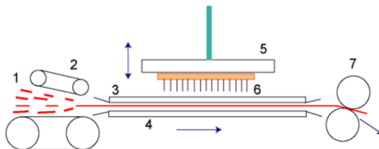
Obrázek 4 Schéma vpichovacího stroje: 1 – vlákná vrstva, 2 – vstupní ústrojí, 3 – stírací rošt, 4 – opěrný rošt, 5 – jehelní deska, 6 – vpichovací jehla, 7 – odváděcí válce [18]
