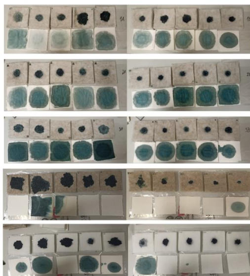
Obrázek 16 Vzorky po nasáknutí 20 ml obarvené kapaliny
