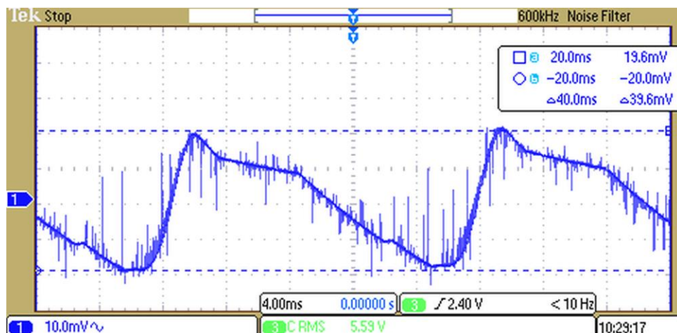
Obr. 7.7-Zvlňenie napätia nábojovej pumpy pri výstupnej frekvencii 51 Hz
