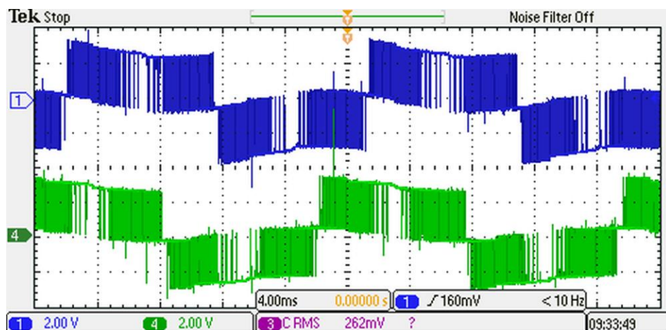
Obr. 7.2-Priebehy výstupných združených napätí
