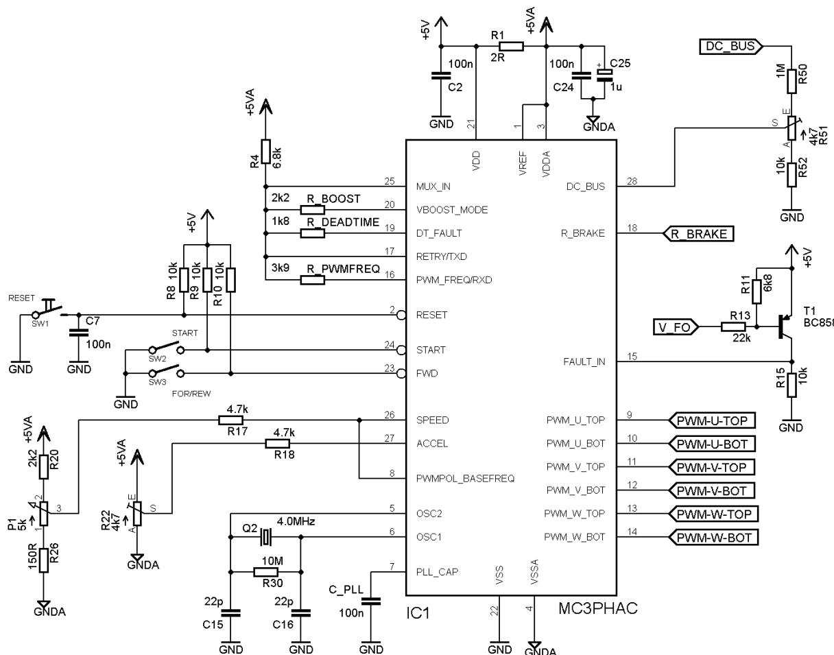
Obr. 4.1-Zapojenie riadiaceho obvodu
