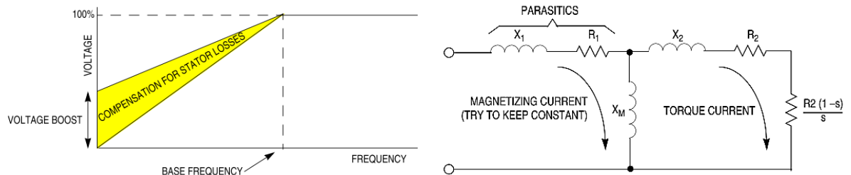
Obr. 3.3-Kompenzácia úbytku napätia v statore [2]
