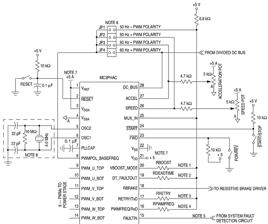
Obr. 3.1-Katalógové zapojenie obvodu MC3PHAC v samostatnom móde [2]
