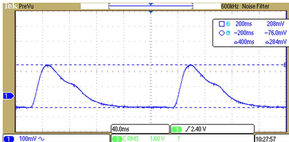
Obr. 7.6-Zvlňnie napätia nábojovej pumpy pri výstupnej frekvencii 5 Hz
