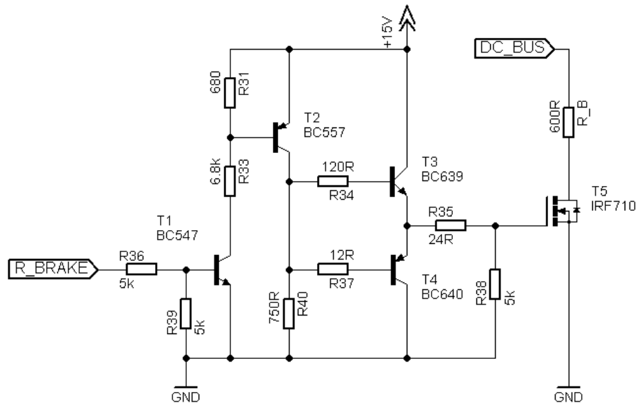
Obr. 4.5-Zapojenie spínača brzdňého odporu
