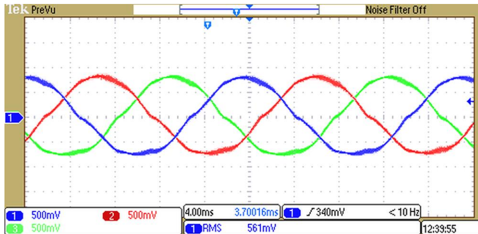
Obr. 7.1-Priebehy výstupných prúdov meniča
