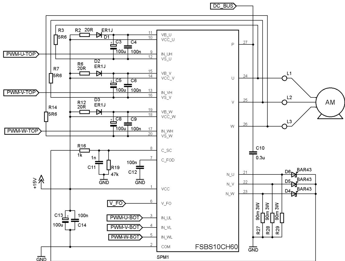
Obr. 4.2-Zapojenie spínacieho modulu
