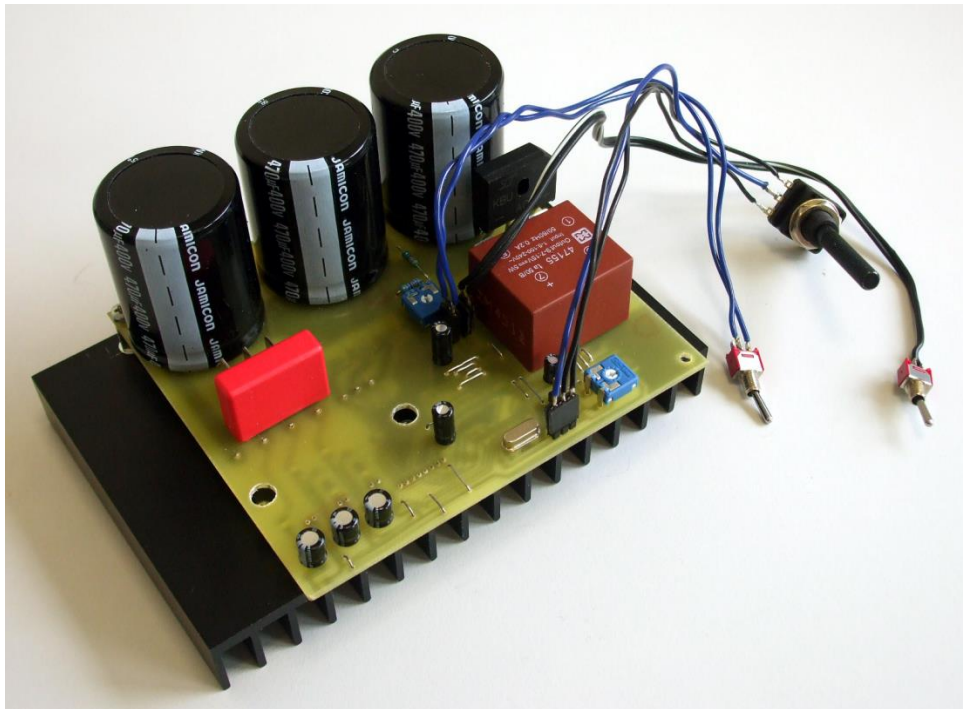
Obr. 6.2-Menič s provizorními ovládacími prvky
