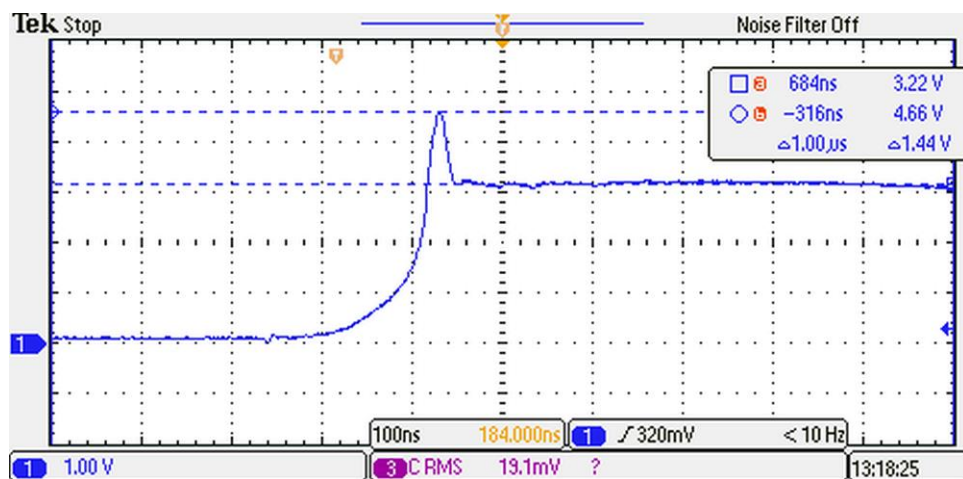
Obr. 7.4-Priebeh napätia na tranzistore pri vypínaní
