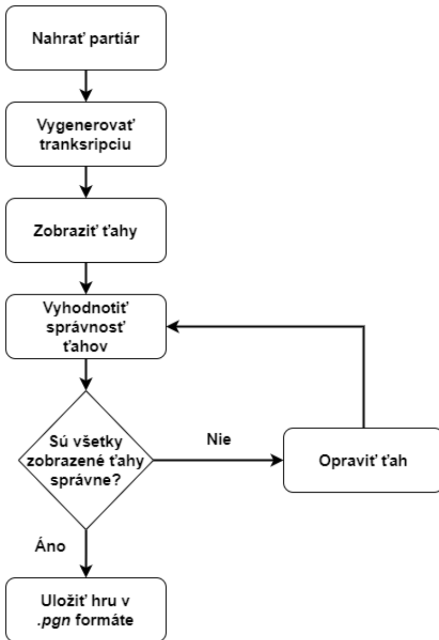
Obr. 5.2: Diagram práce uživateľa so systémom.
