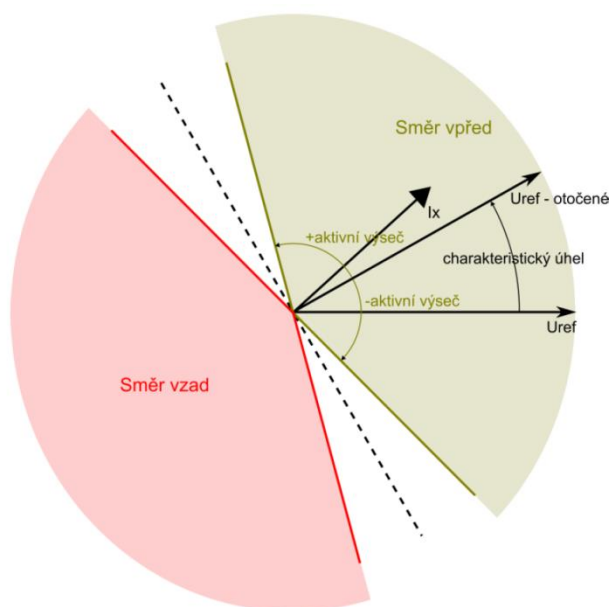
Obr. 5-8 Směrová charakteristika [14]
