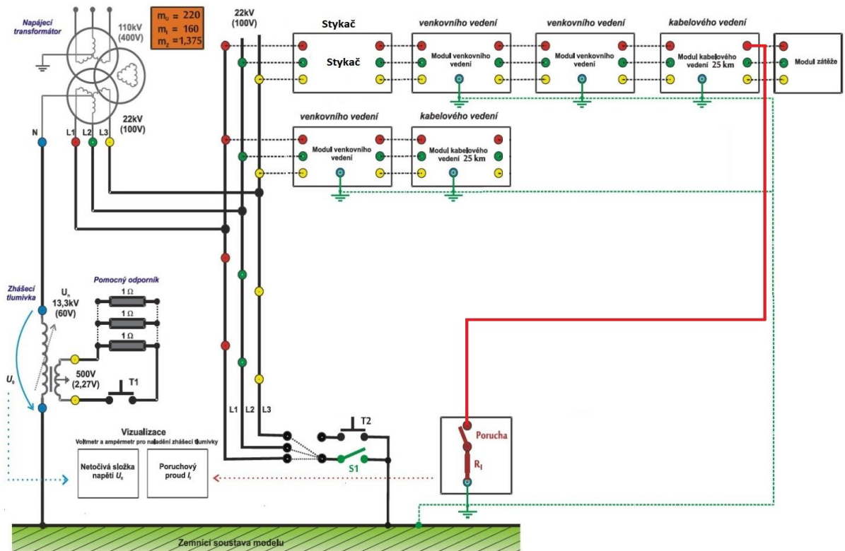
Obr. 8-9 Schéma poruchy
