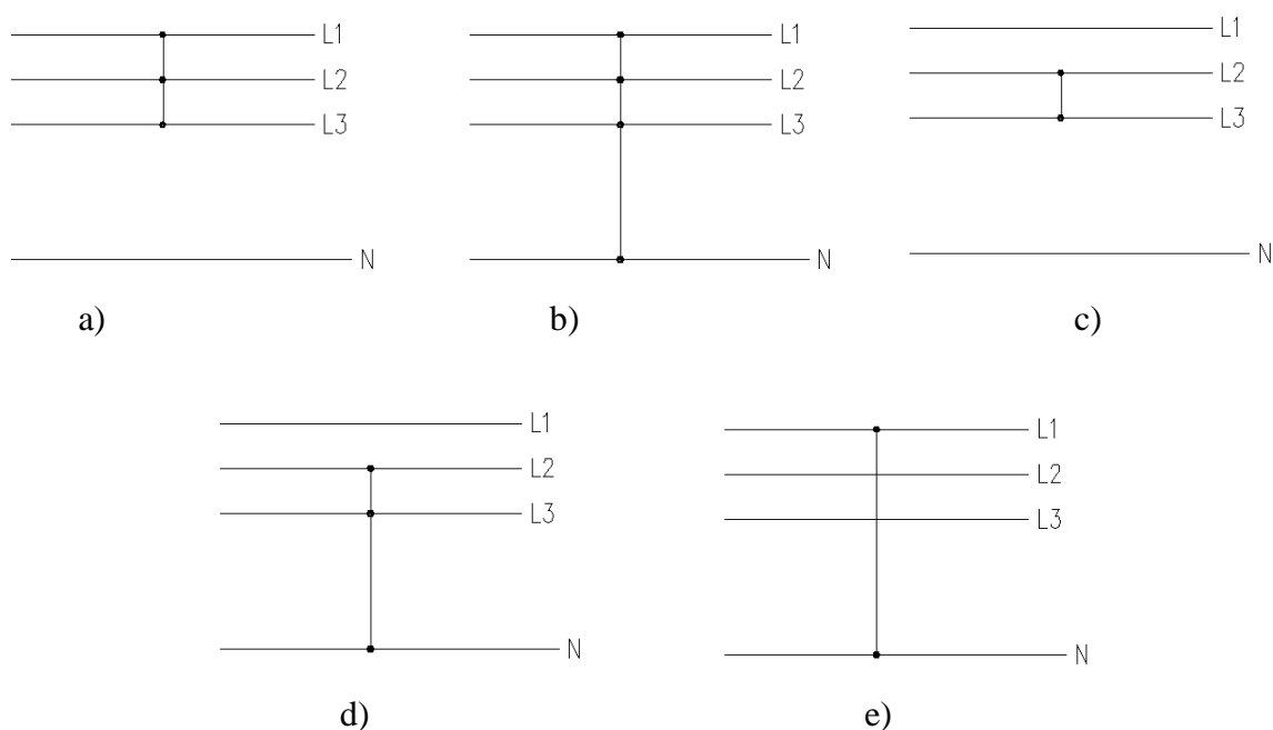
Obr. 2-1 Druhy zkratů [3]
