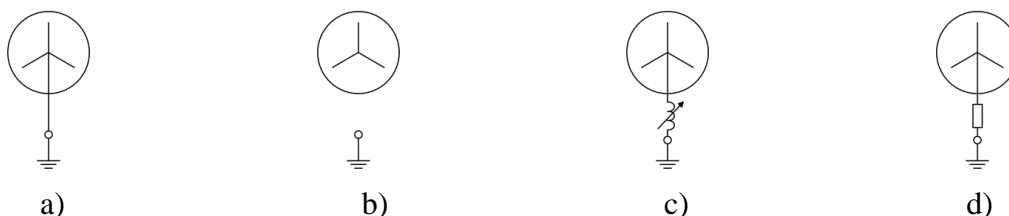
Obr. 1-2 Příklady možných způsobů uzemnění nulového bodu soustavy. [1]
