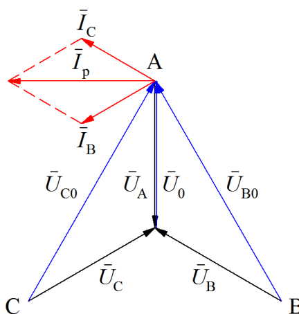
Obr. 3-2 Fázorový diagram pro zemní spojení v bodě A [1]
