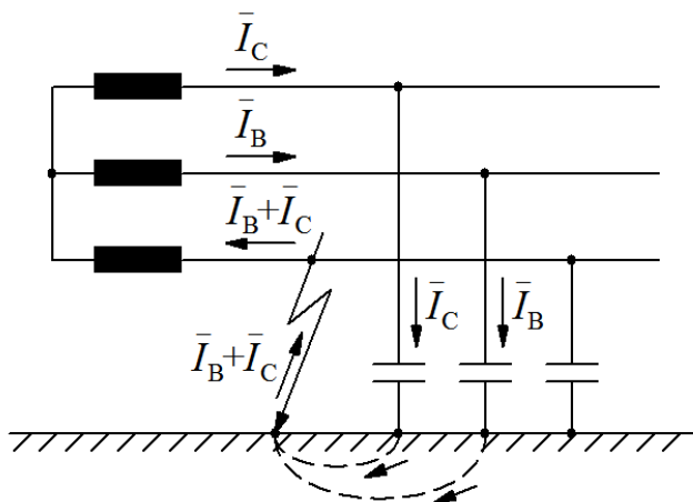
Obr. 3-1 Schématické znázornění sítě s izolovaným uzlem při zemním spojení [1]
