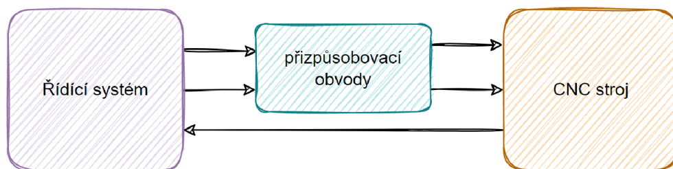
Obr. 3 Zjednodušené blokové schéma obráběcího stroje s číslíkovým řízením (zdroj: Barčík 2009)
