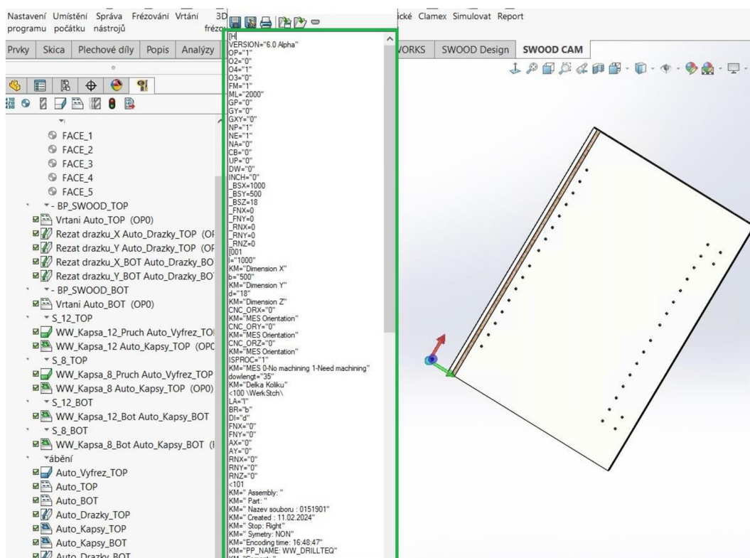
Obr. 55 Vygenerovaný NC program pro dílec vyobrazený v SolidWorks s pomocí Swood CAM (zdroj: autor)
