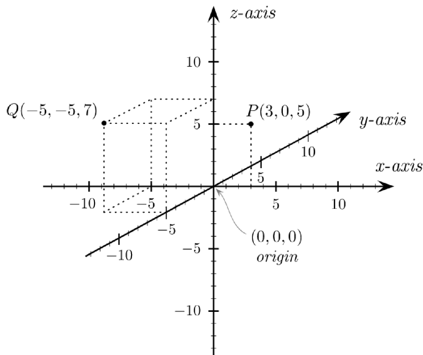
Obr. 10 Kartézské souřadnice s body v 3D prostoru (zdroj: wikimedia.org [online]. [cit. 31.3.2023])
