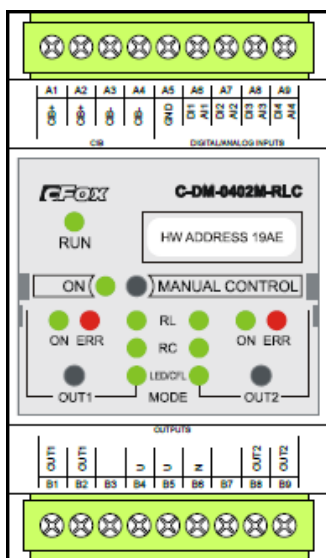
Obr. 4-7 Stmívací modul C-DM-0402-RLC [12]
