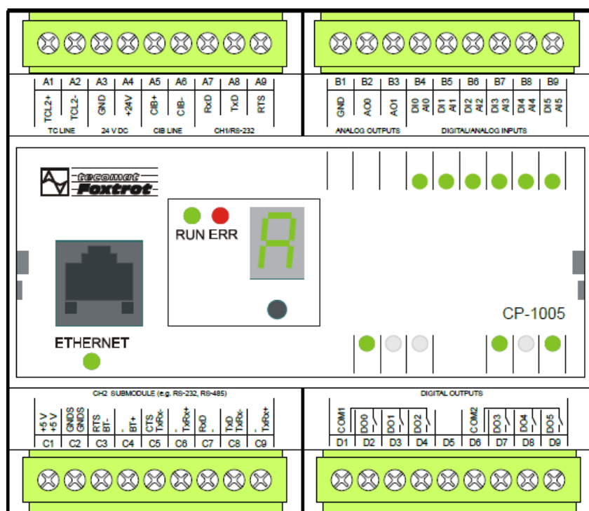
Obr. 4-1 Základní modulo CP-1005 [12]
