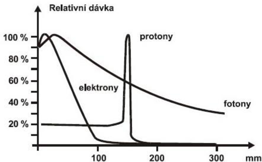
Obrázek 8 - Srovnání dávky záření v závislosti na hloubce, zdroj: Šlampa, 2012
