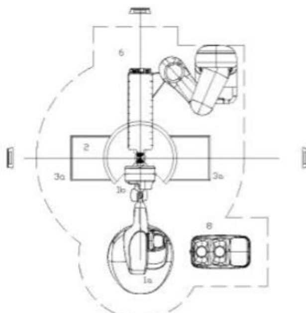
Obrázek 15 - Půdorys rozvržení komponentů, zdroj: Oberstein
