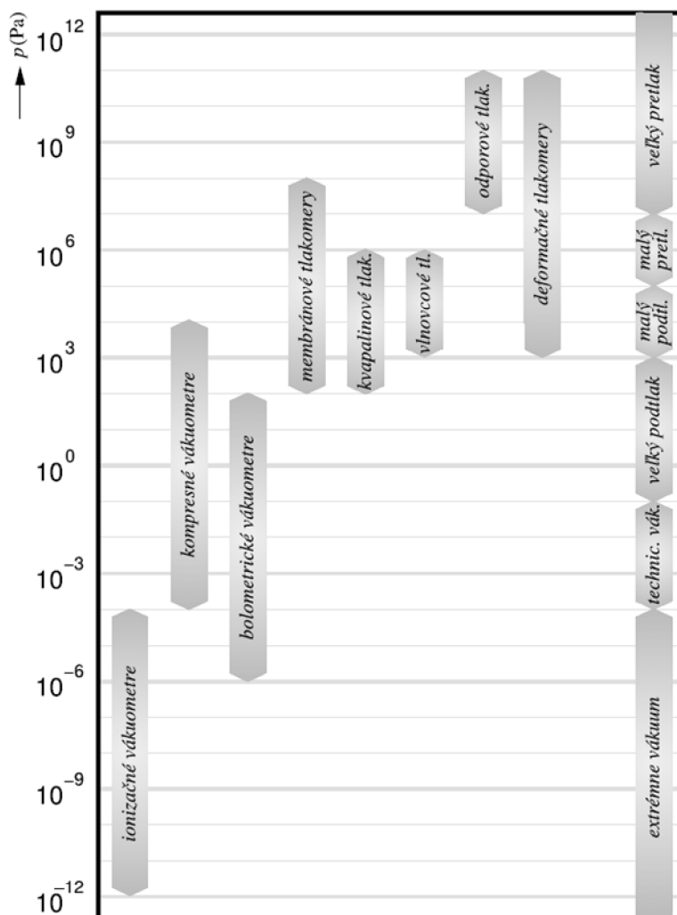
Obr. 10 Rozdelenie tlakomerov podľa ich meracieho rozsahu [18]
