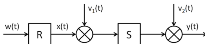
Obr. 1 Schéma ovládania
