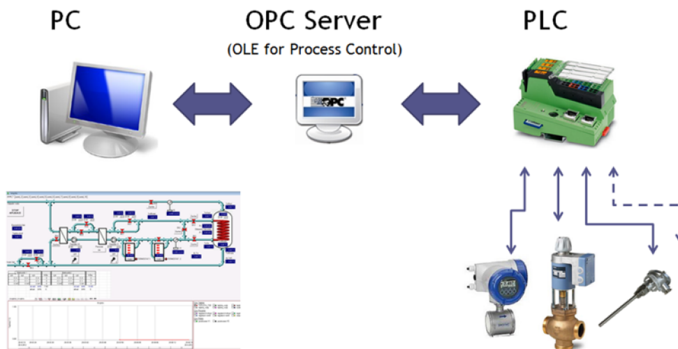
Obr. 34 Architektúra riadenia hydraulickej slučky
