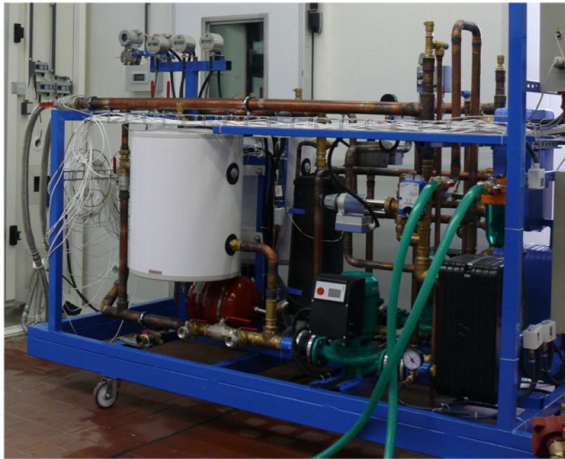
Obr. 16 Hydraulická slučka v Strojárskeho zkušebnom ústavu, s.p.,
