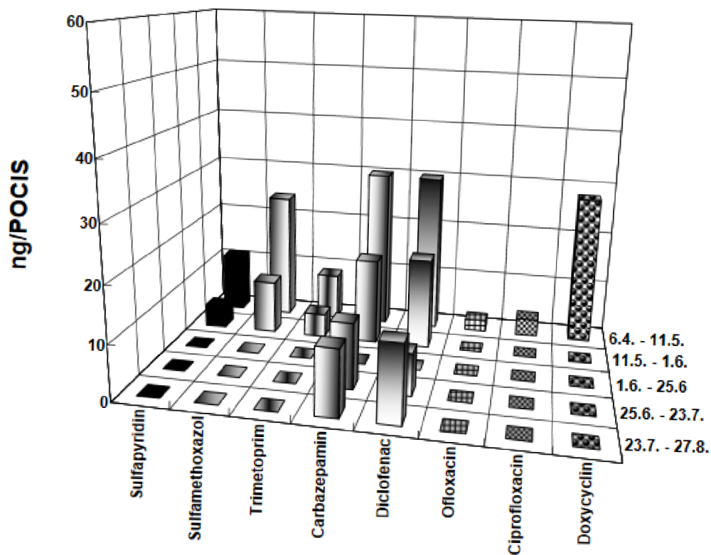
Obr. 7. 4 Koncentrace léčiv po sedimentaci a filtraci [36]
