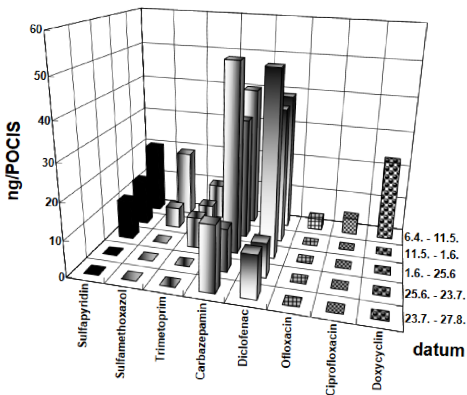
Obr. 7. 3 Koncentrace léčiv v surové vodě [36]
