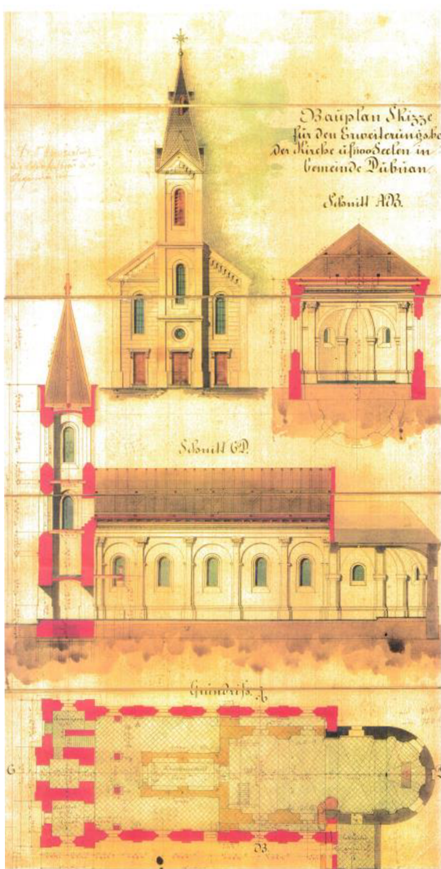
Příloha č. 5 Stavební plán kostela v Dubňanech
