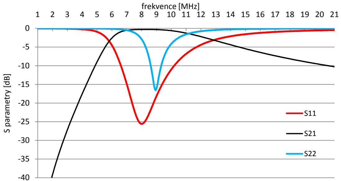
Obrázek 3.21 Simulované parametry pásmové propusti 9MHz.
