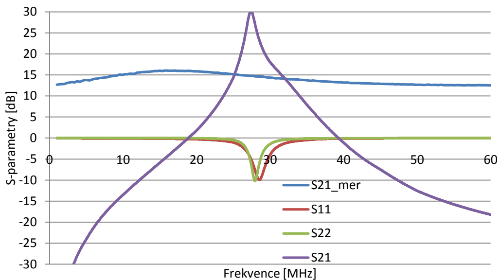
Obrázek 3.5 S-parametry přízpusobeného LNA.
