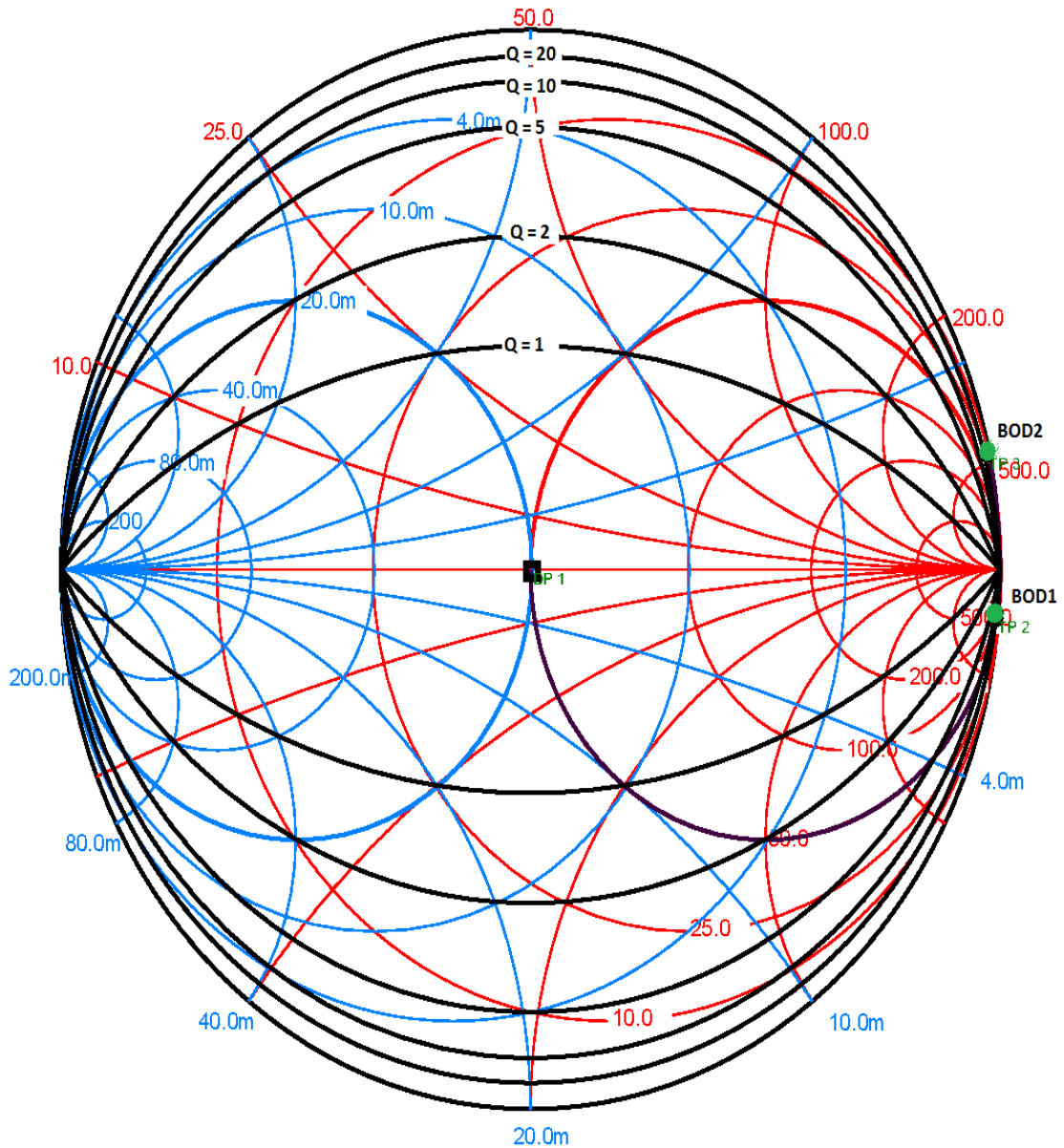
Obrázek 2.16 Smithův diagram s kružnicemi konstantní jakosti obvodu.
