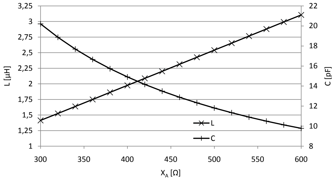
Obrázek 2.7 Rozptyl hodnot indukčnosti a kapacity v závislosti na reaktanci.
