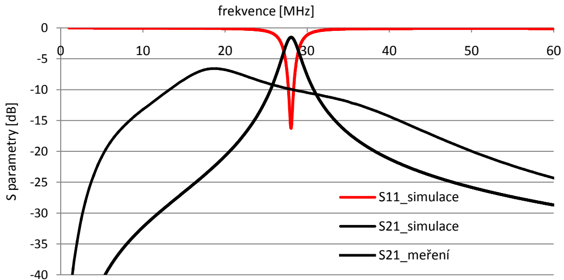
Obrázek 3.11 Měření přenosu pásmové propusti 28 MHz.
