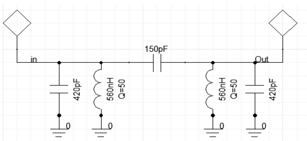
Obrázek 3.20 Schéma zapojení pásmové propusti 9 MHz.
