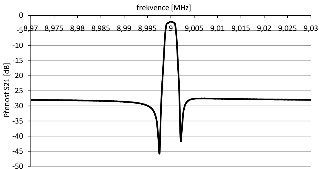
Obrázek 3.17 Přenos selektivní pásmové propusti.
