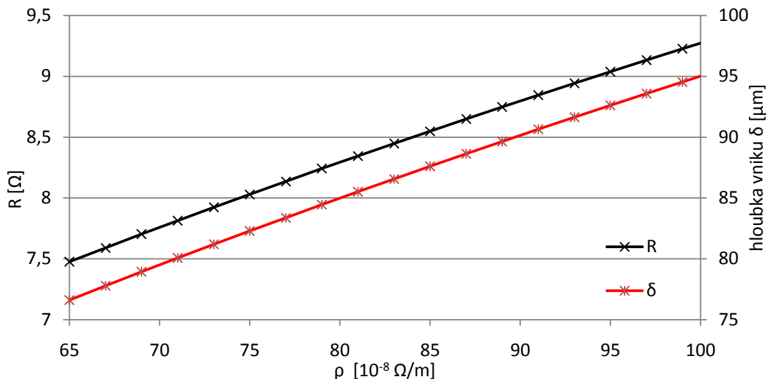
Obrázek 2.2 Závislost odporu pro střídavý proud na rezistivitě.
