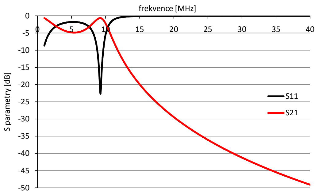
Obrázek 3.36 Přenosová charakteristika pro oscilátor na 9 MHz.
