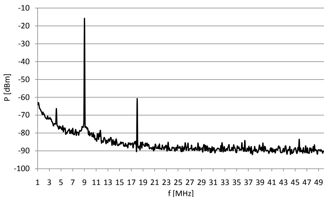
Obrázek 3.38 Změřené spektrum oscilátoru 9 MHz.
