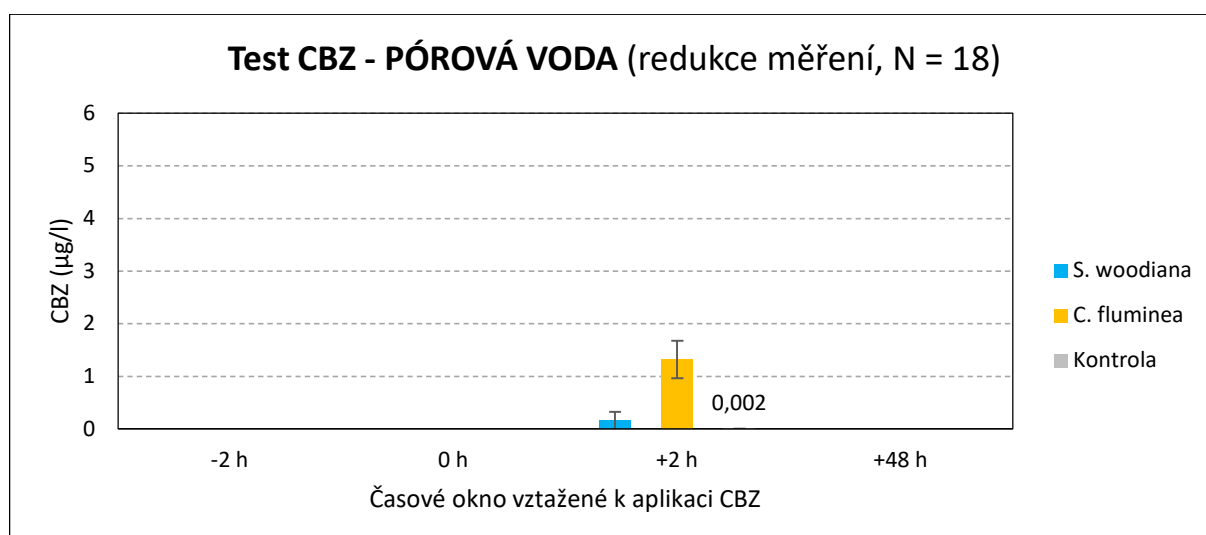
Obr. 20. Hodnoty karbamazepinu (CBZ) (vyjádřené jako průměr ± SD) v pórové vodě v závislosti na času a typu kádinky (test CBZ, redukovaná data)
