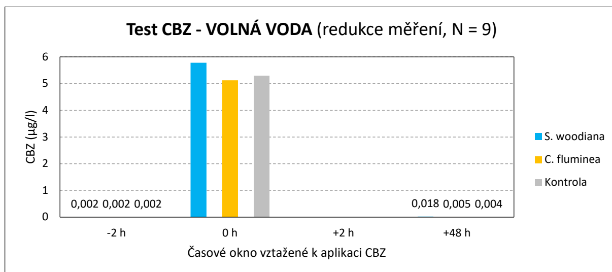
Obr. 19. Hodnoty karbamazepinu (CBZ) ve volné vodě v závislosti na času a typu kádinky (test CBZ, redukovaná data)
