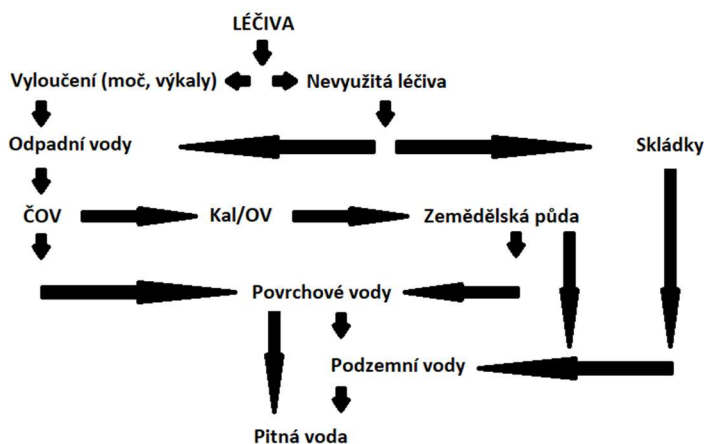
Obr. 2. Osud léčiv v prostředí (OV = odpadní vody) (autor: Vojtěch Barák; upraveno dle Halling-Sørensen et al. 1998)
