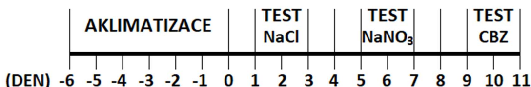
Obr. 8. Časová osa znázorňující průběh experimentu
