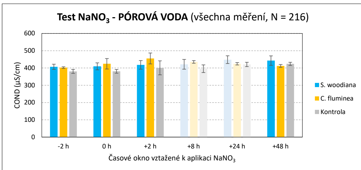
Obr. 14. Hodnoty konduktivity (vyjádřené jako průměr ± SD) v pórové vodě v závislosti na času a typu kádinky (test NaNO 3 )
