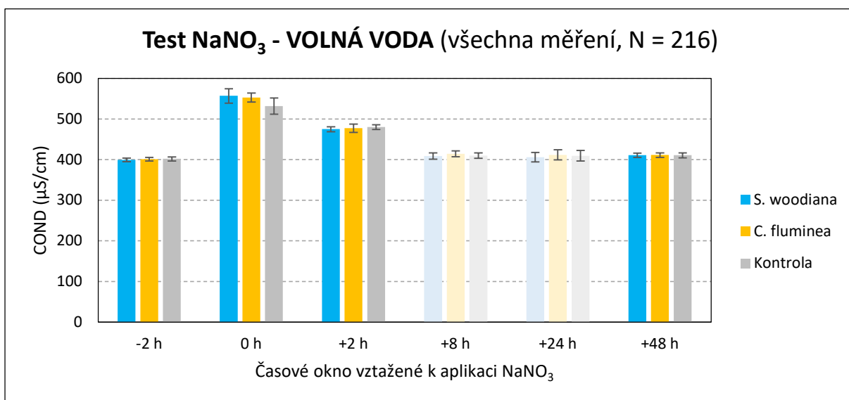
Obr. 13. Hodnoty konduktivity (vyjádřené jako průměr ± SD) ve volné vodě v závislosti na času a typu kádinky (test NaNO 3 )
