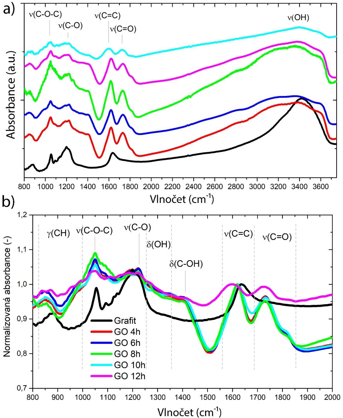
Obrázek 19: a) FTIR spektrum pro grafit a GO po 4, 6, 8, 10 a 12 hod. oxidace od vlnočtu 800–3750 cm -1 (legenda stejná jako u grafu b). b) Normalizované FTIR spektrum pro grafit a GO po 4, 6, 8, 10 a 12 hod. oxidace od vlnočtu 800–2000 cm -1 .
