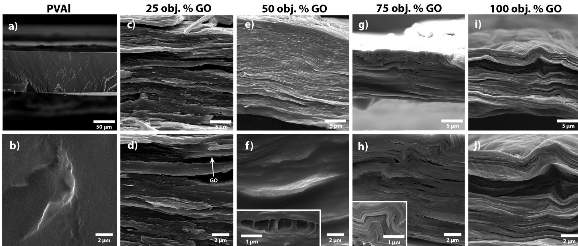
Obrázek 21: SEM snímky a), b) PVAI filmu; c), d) PVAI/GO nanokompozitu s 25 obj % GO; e), f) PVAI/GO nanokompozitu s 50 obj % GO s detailem na dutinu přemostěnou vláknou PVAI; g), h) PVAI/GO nanokompozitu s 75 obj % GO s detailem na vrstevnatou strukturu; i), j) filmu tvořeného 100 % GO.
