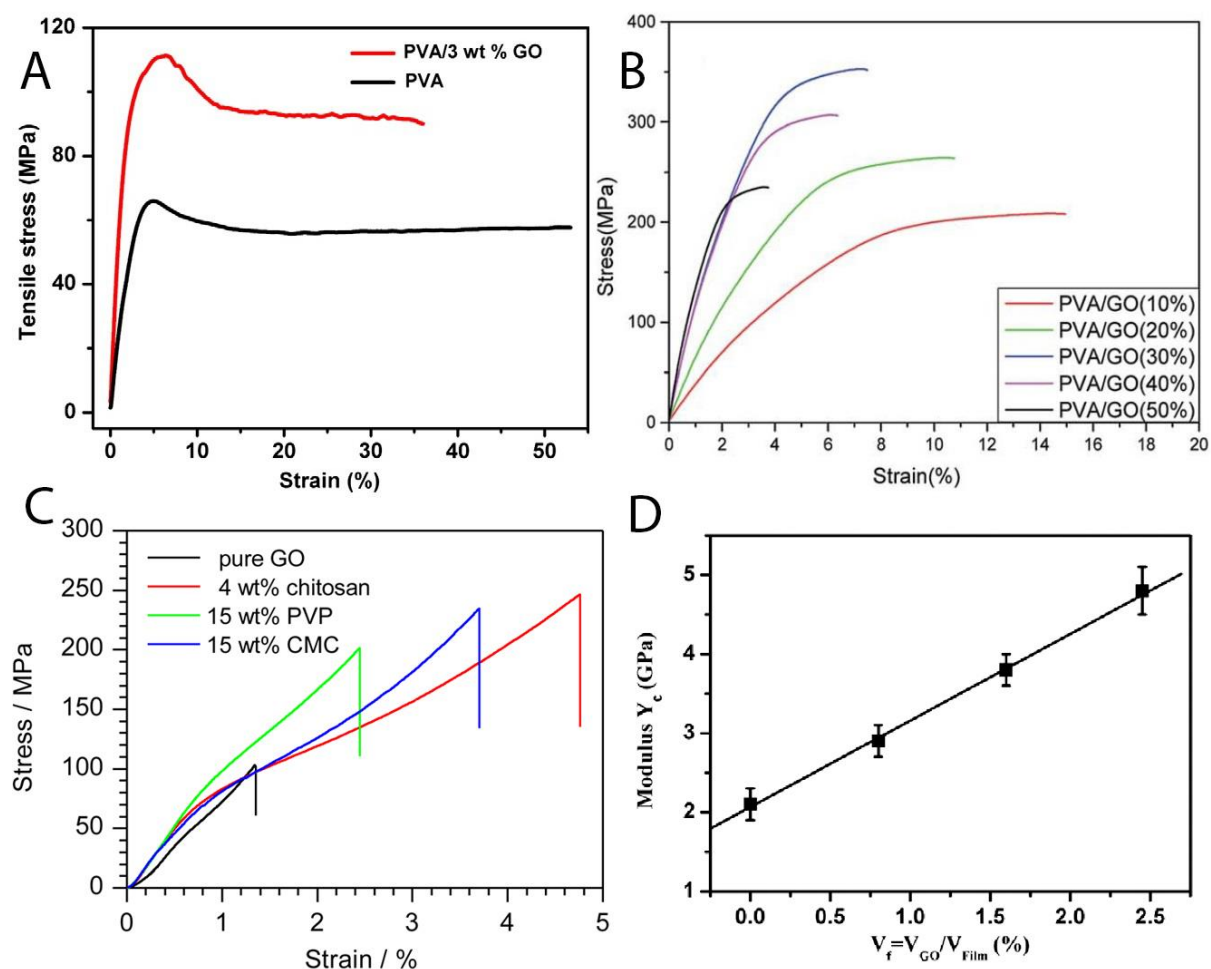
Obrázek 9: Porovnání závislosti napětí v tahu (Tensile stress/Stress) na prodloužení (Strain) pro a) PVAI a PVAI/GO kompozit s 3 hm. % GO [39], b) pro nanokompozit PVAI/GO s obsahy GO 10–50 % [40], c) pro čistý GO (pure GO), nanokompozit obsahující 4 hm. % chitosanu, 15 % PVP a 15 % karboxymethylcelulózy (CMC) [41]. d) Závislost Youngova modulu pružnosti na objemovém zlomku GO v PVA matici [39].
