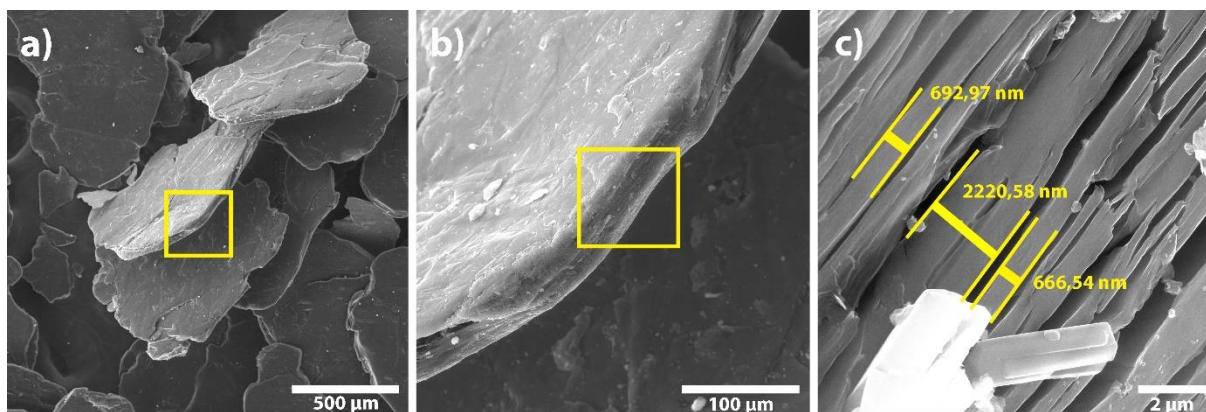
Obrázek 15: a) SEM snímek grafitu. b) Detail zvýrazněné oblasti strany jedné částice grafitu. c) Detailní přiblížení zvýrazněné oblasti s velikostmi jednotlivých vrstev grafitu.
