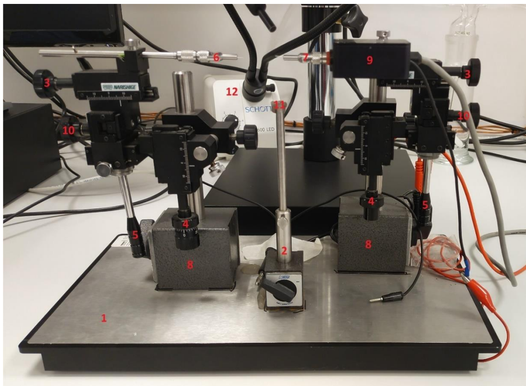
Obrázek 8. Elektroantenograf (EAG)
