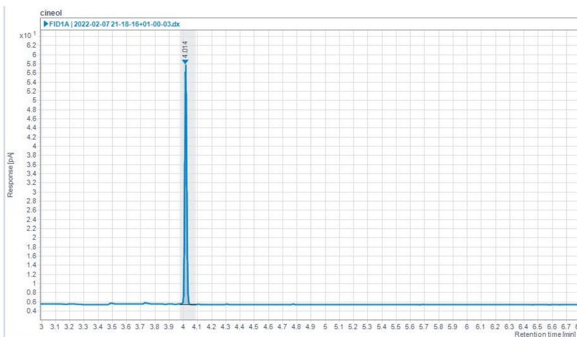
Graf 3 – Detail GC-MS analýzy 1,8-cineolu
