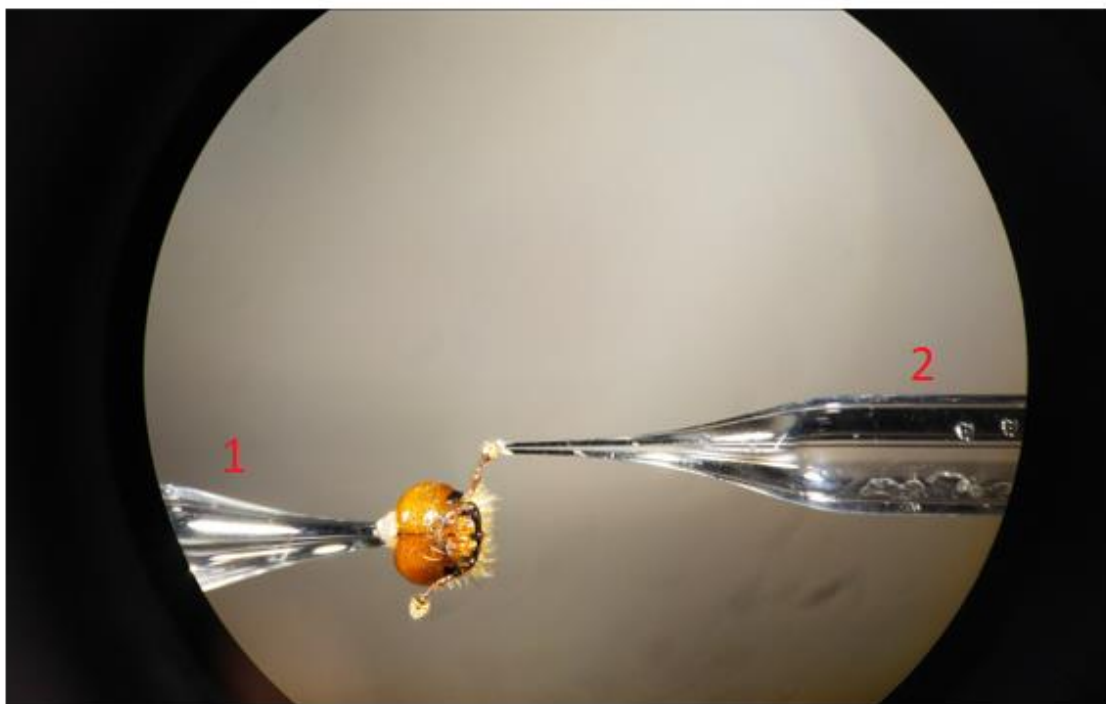
Obrázek 9. Detailní pohled pod mikroskopem na fixaci hlavy lýkožrouta smrkového 1 = referenční elektroda, 2 = měřící elektroda.
