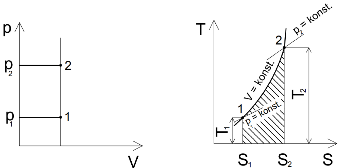
Obr. 2 Izochorická komprese v p-V a T-s diagramu.
