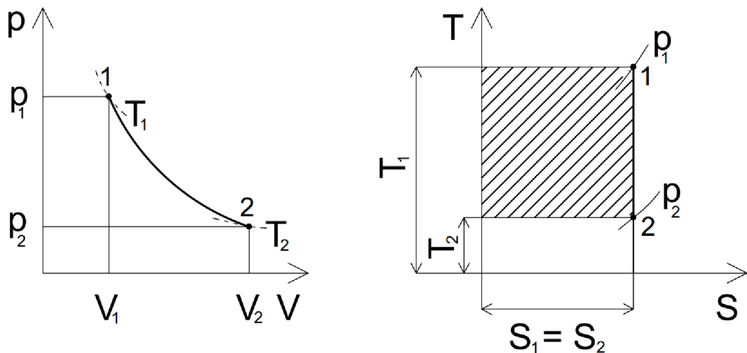
Obr. 4 Adiabatická expanze v p-V a T-s diagramu.
