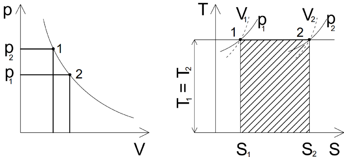
Obr. 3 Izotermická expanze v p-V a T-s diagramu.
