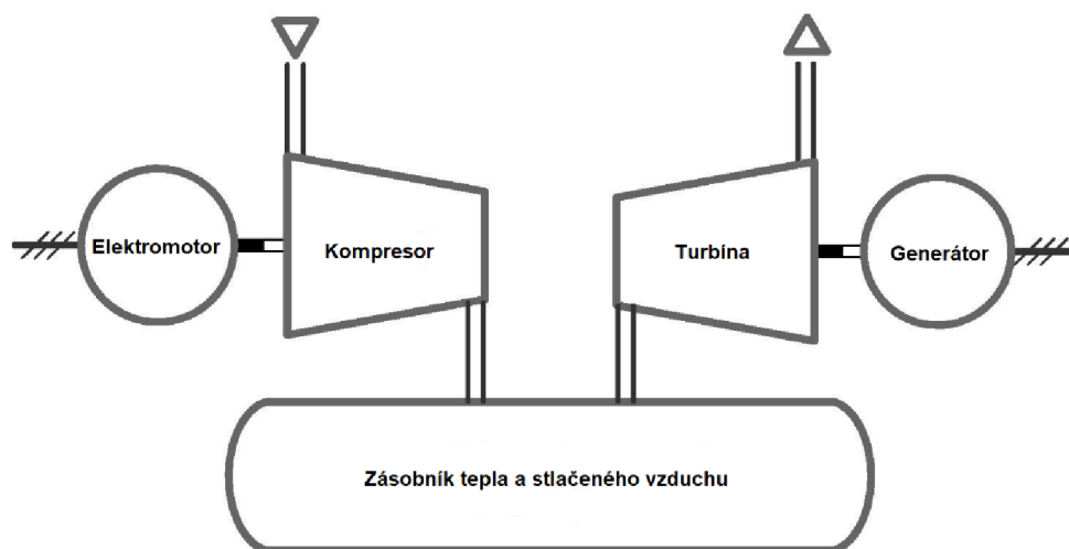
Obr. 12 Schéma CAES bez systému TES, upraveno dle [20].
