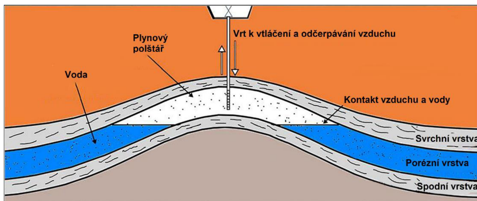
Obr. 8 Schéma akviféru, upraveno dle [15].
