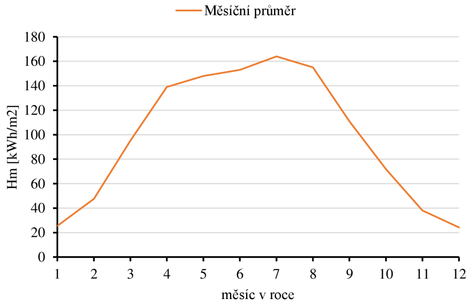
Roční úhrn solárního záření na nakloněné rovině
