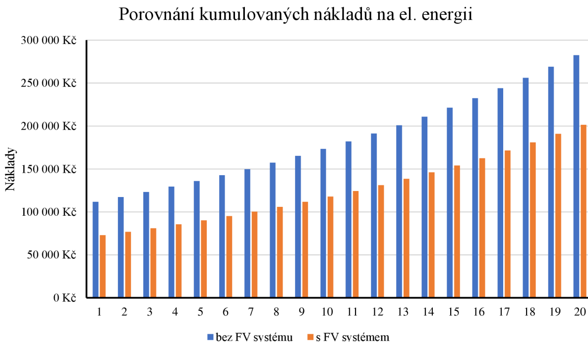
Obr. 9-2 Porovnání nákladů na el. energii
