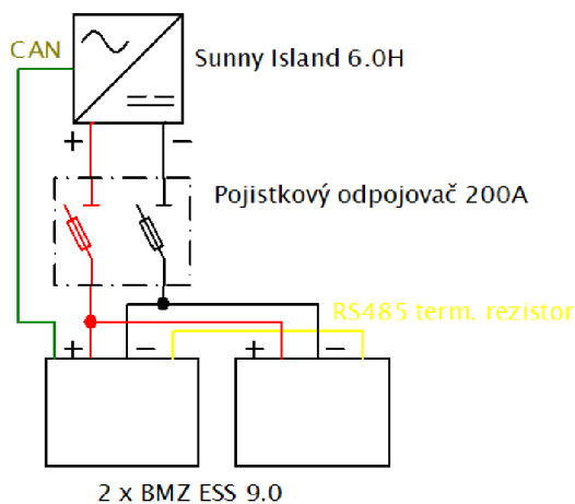
Obr. 7-10 Schéma připojení bateriového systému
