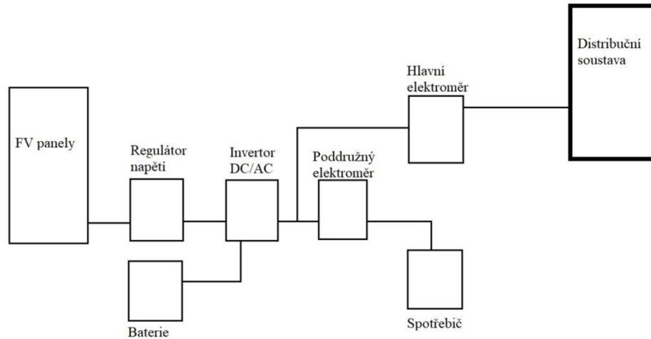
Obr. 2-7 Hybridní systém
