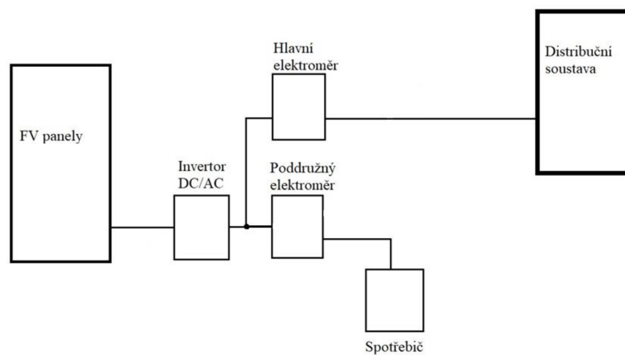
Obr. 2-8 Distribuční systémy
