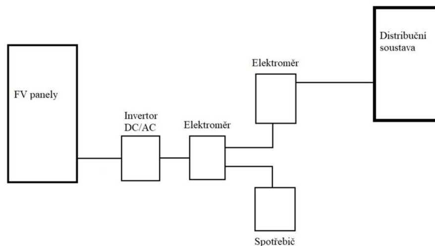
Obr. 2-6 Spotřebitelský systém
