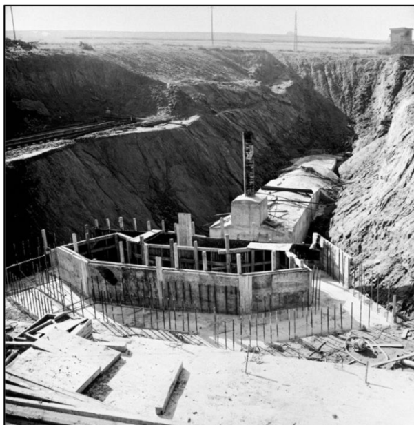
Obrázek 3: Začátek štolového přivaděče (Aktuálně, 2022).
