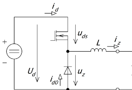
Obr. 3.2 Snižující měnič, převzato z [9]
