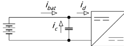
Obr. 4.10 Principiální schéma s vyznačenými směry proudů
