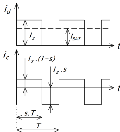
Obr. 4.11 Idealizované průběhy proudů i_d(t) a i_c(t)
