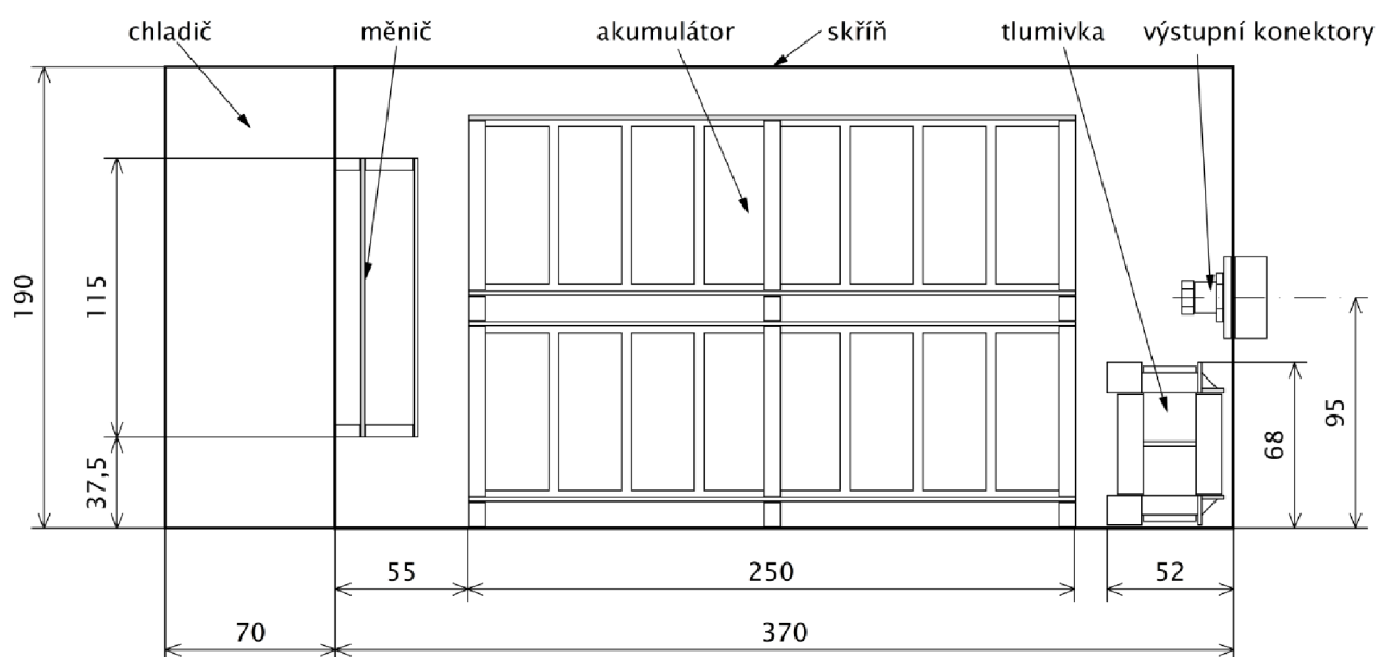
Obr. 7.1 Náčrt prostorového rozvržení svářečky
