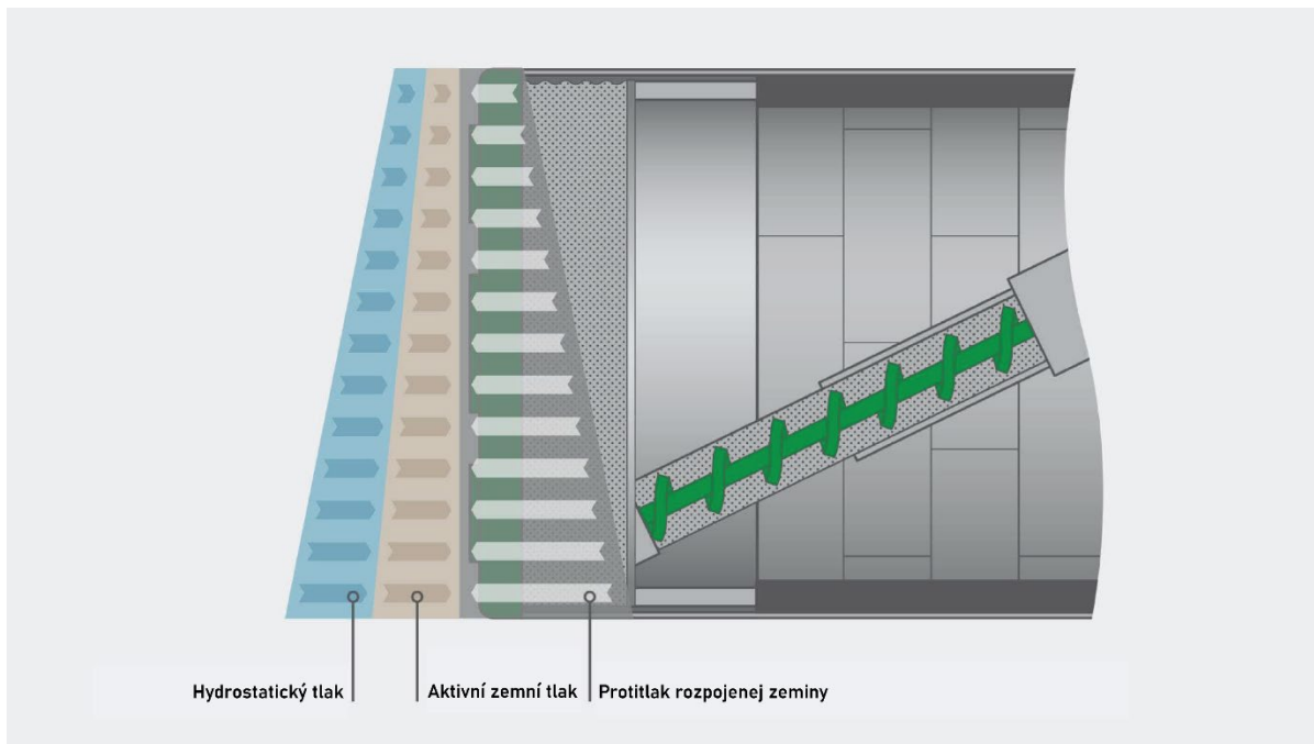
Obr. 7 Funkce zeminového štítu (11)
