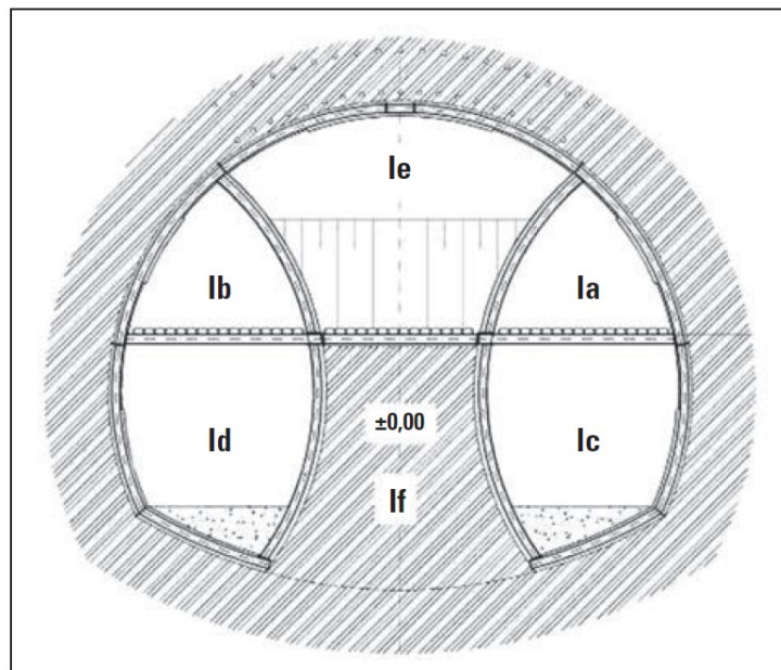
Obr. 9 Rozdělení výrubu (11)
