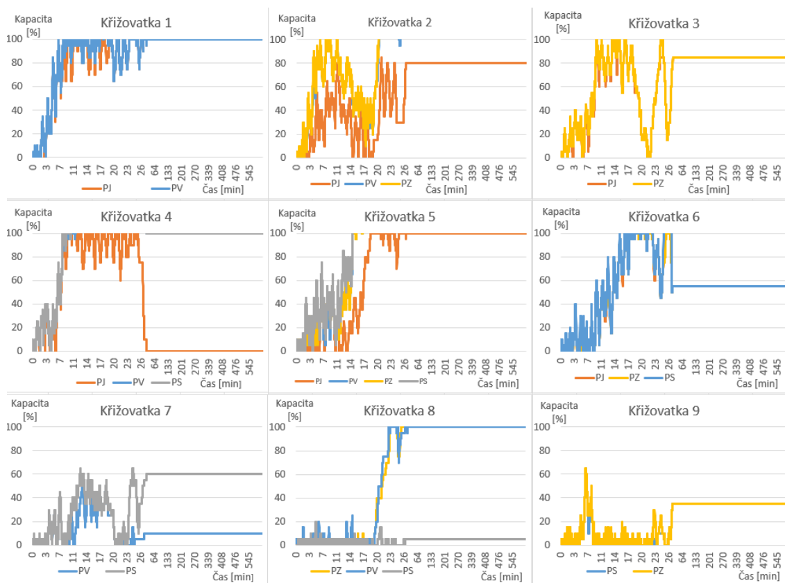
Graf 4: Napnění kapacity příjezdových cest v čase
