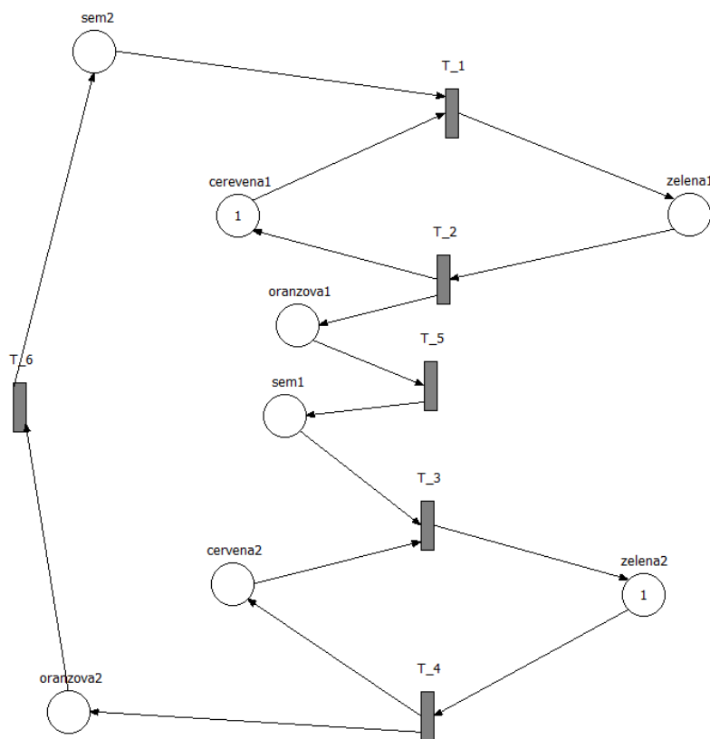
Obrázek 10: Schéma semaforu
