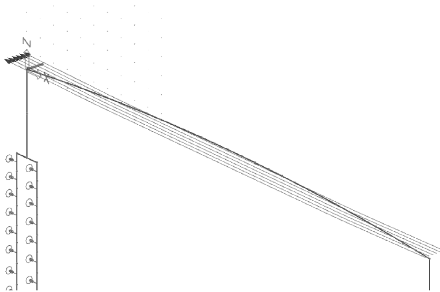
Obrázek 15 - Model kabelů v programu Scia Engineer
