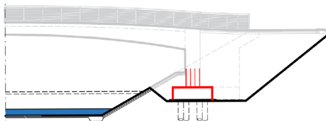
Obrázek 37 - Fáze výstavby 5
