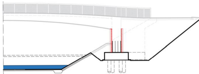
Obrázek 38 - Fáze výstavby 6
