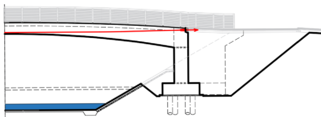
Obrázek 42 - Fáze výstavby 10
