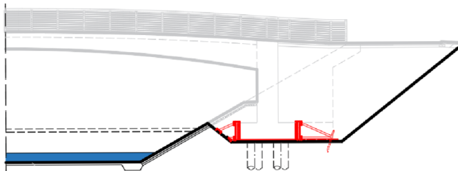
Obrázek 36 - Fáze výstavby 4
