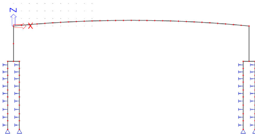
Obrázek 10 - Podepření modelu
