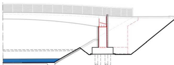
Obrázek 39 - Fáze výstavby 7
