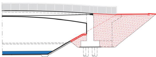
Obrázek 43 - Fáze výstavby 11
