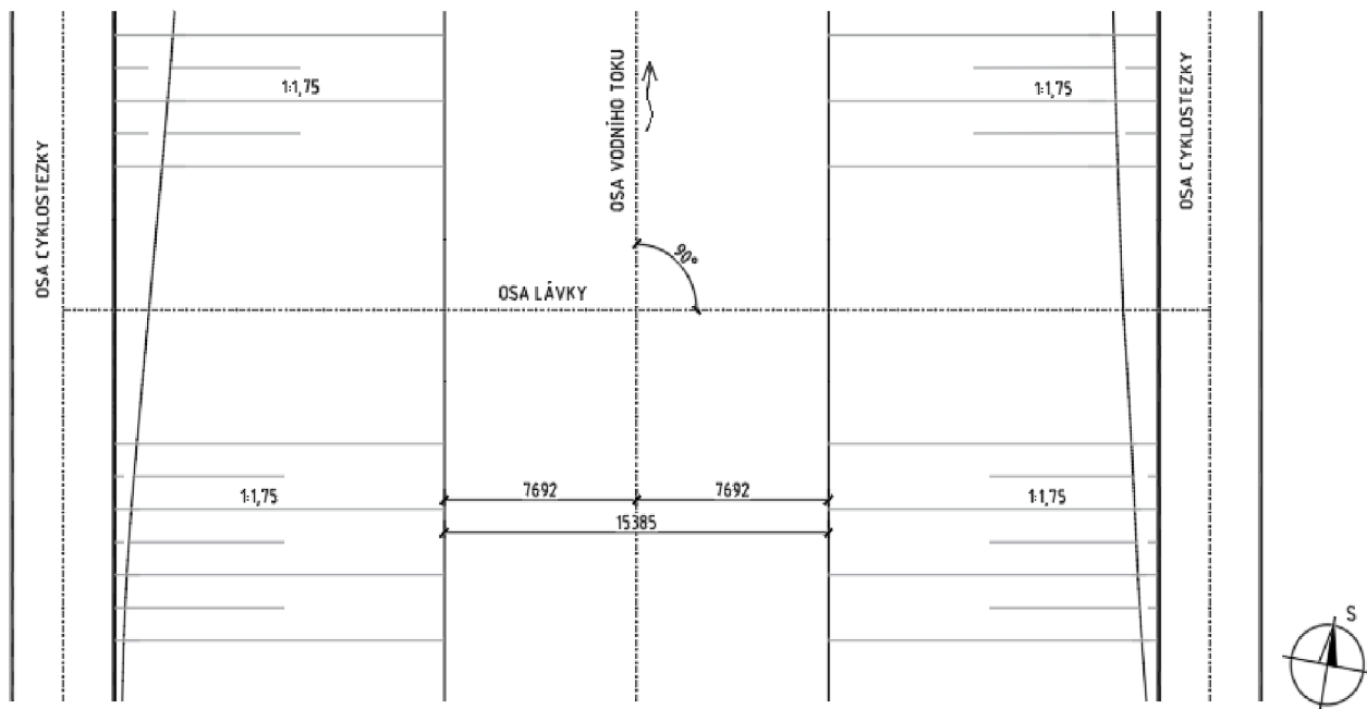
Obrázek 1 - Situace v předpokládaném místě křížení
