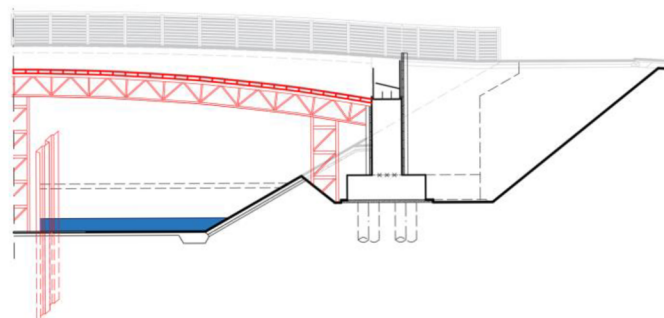
Obrázek 40 - Fáze výstavby 8
