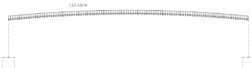
Obrázek 19 - Ostatní stálé zatížení
