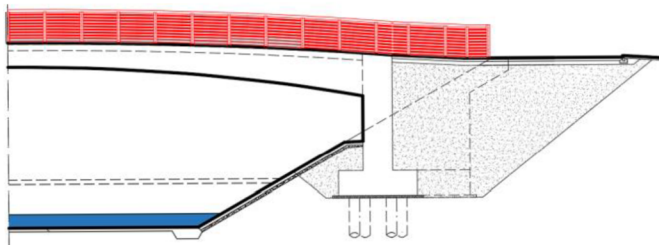
Obrázek 44 - Fáze výstavby 12
