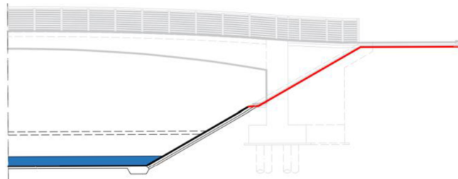
Obrázek 34 - Fáze výstavby 2
