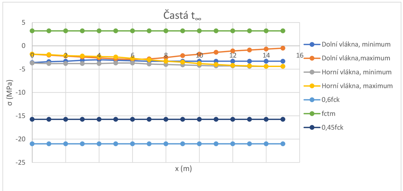
Obrázek 27 - Graf napětí v čase t_{\infty} - častá kombinace
