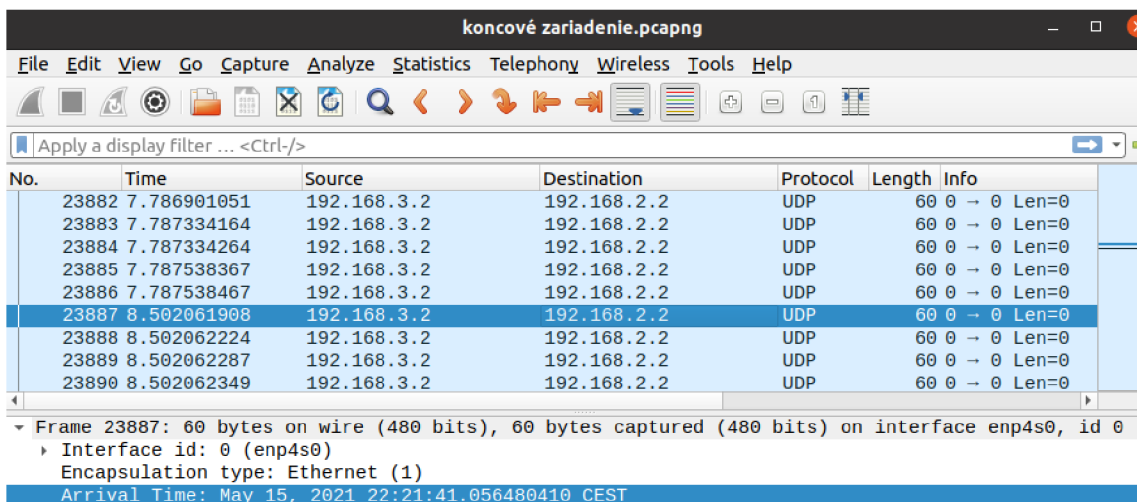
Obr. 5.7: Wireshark na koncovom zariadení
