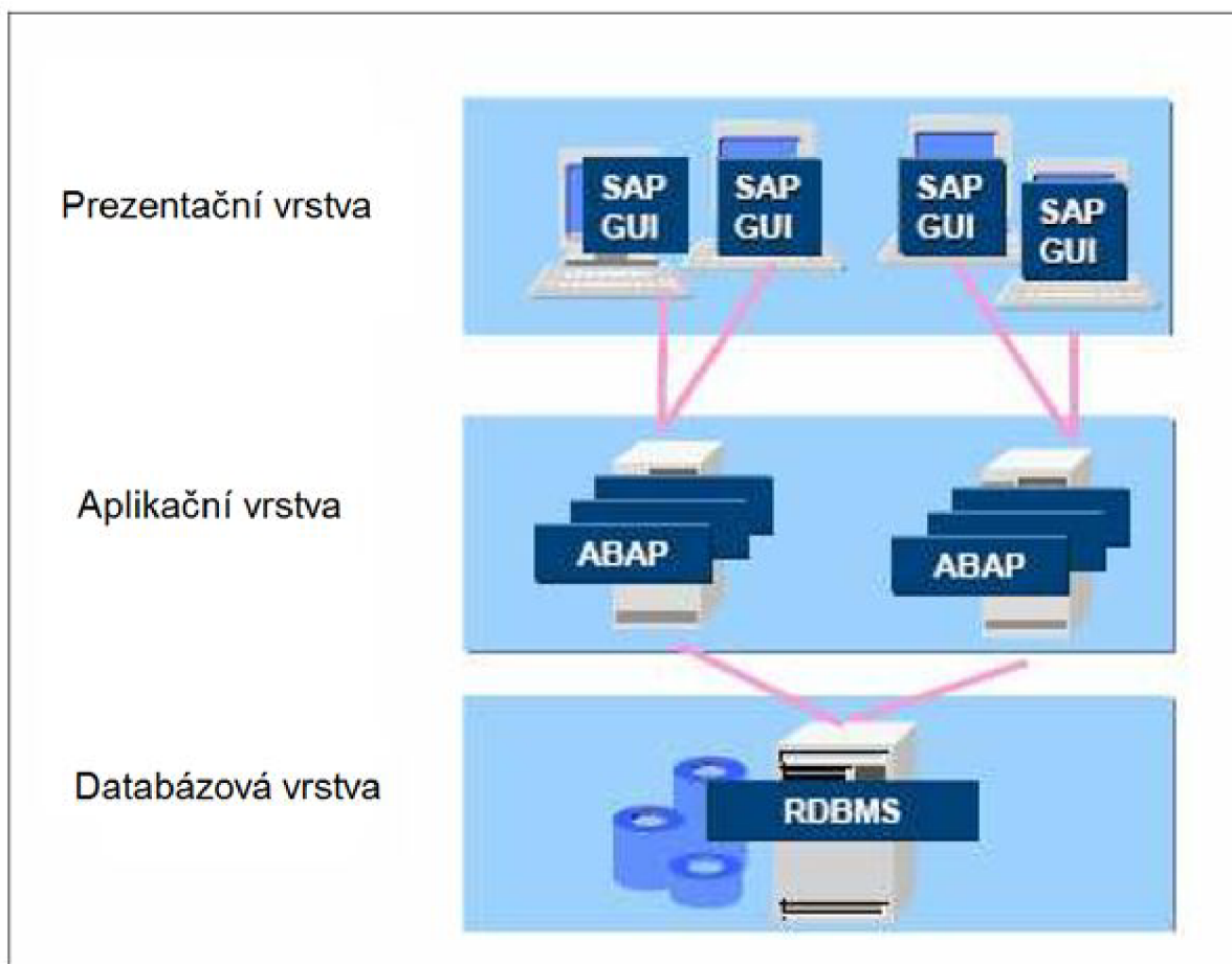
Obrázek 2.2: Architektura systému [5]
