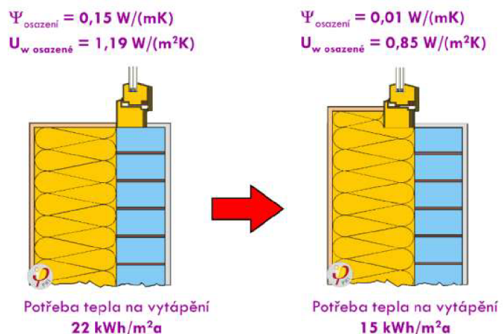
Obrázek 4 - Vliv osazení okna na tepelné ztráty objektu [13]
