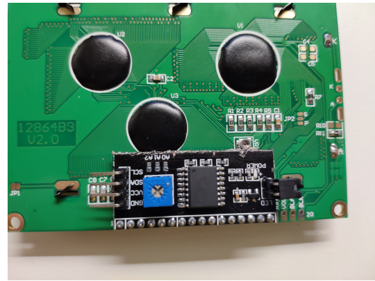
Obr. 3.10: Převodník PCF8574
