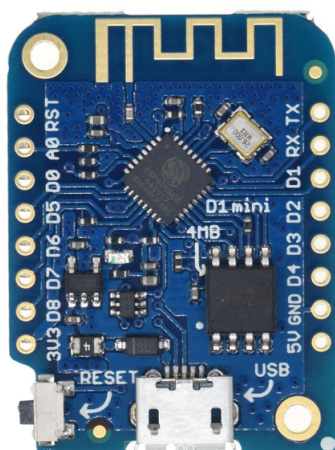
Obr. 3.1: Modul Wemos D1 mini [17]
