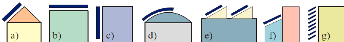
Obr. 2.7.1: Schematické znázornění způsobů integrace FV systémů do budov: (a) šikmá střecha, (b) plochá střecha, (c) fasáda, (d) tenkovrstvá FV pro velké střešní plochy, (e) průmyslové aplikace, (f) semitrparentní FV pro atria a výplně otvorů, (g) vnější stínící a clonící systémy [2]
